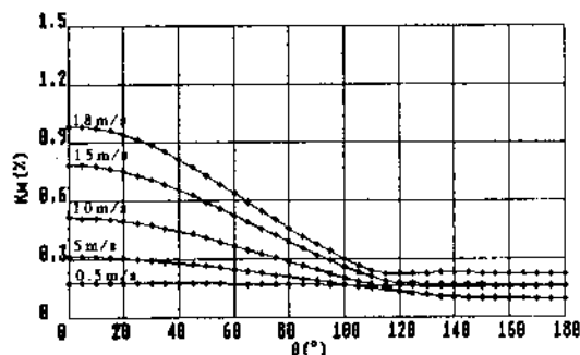
Sl. 19 Koeficijent smanjenja verovatnoće pogađanja u funkciji intenziteta i napadnog ugla vetra za potkalibarnu municiju; Wr=0,5 do 18 \text{ m/s} ; Vt=25 \text{ km/h} ; tv=-30^\circ\text{C} ; X=2000 \text{ m}
