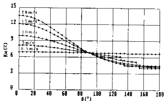
Sl. 24 Koeficijent smanjenja verovatnoće pogadjanja u funkciji intenziteta i napadnog ugla vetra za kumulativnu municiju prema predlogu novih granica; W_r=0,5\text{ do }18\text{ m/s} ; V_t=25\text{ m/s} ; t_v=-30^{\circ}\text{C} ; X=2000\text{ m}
