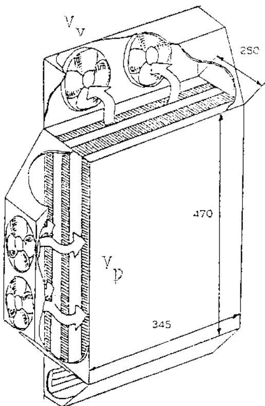
Sl. 9 Slaganje termoelektričnih elemenata
