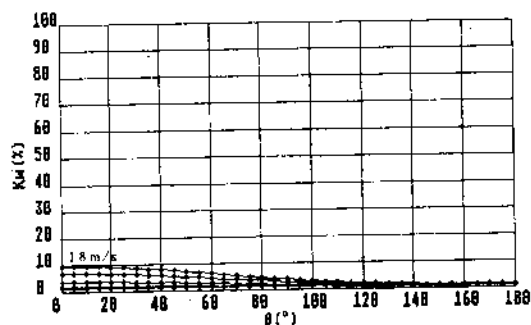
Sl. 17 Koeficijent smanjenja verovatnoće pogađanja u funkciji intenziteta i napadnog ugla vetra za trenutno-fugasnu municiju; Wr=0,5 do 18 \text{ m/s} ; Vt=25 \text{ km/h} ; tv=15,9^\circ\text{C} ; X=2000 \text{ m}
