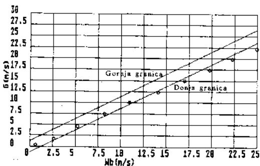
Sl. 7 Rezultati merenja bočne komponente vetra ako je ugao \beta=0^\circ ; t_v=21^\circ\text{C} ; p_v=996,5 mbar
