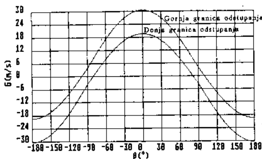
Sl. 6 Gornja i donja granica dozvoljenih maksimalnih odstupanja merenih vrednosti bočnog vetra meteosenzorom u funkciji napadnog ugla kod W_r = 25 \text{ m/s}; t_v = -30^\circ\text{C}
