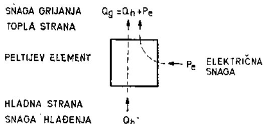
Sl. 2 Učink električne toplotne pumpe
