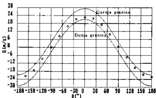
Sl. 8 Rezultati merenja bočne komponente vetra pri variranju ugla \beta W_r=25 m/s; t_v=25^\circ\text{C} ; p_v=998,5 mbar
