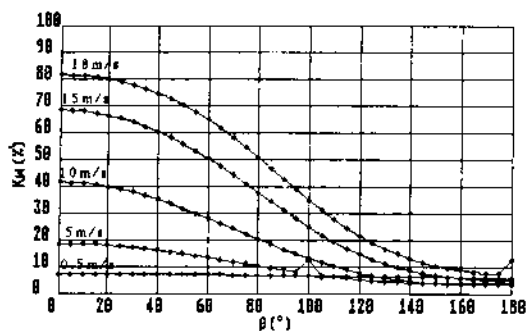
Sl. 15 Koeficijent smanjenja verovatnoće pogađanja u funkciji intenziteta i napadnog ugla vetra za kumulativnu municiju; Wr=0,5 do 18 \text{ m/s} ; Vt=25 \text{ km/h} ; tv=15,9^\circ\text{C} ; X=2000 \text{ m}
