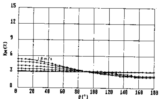
Sl. 23 Koeficijent smanjenja verovatnoće pogadjanja u funkciji intenziteta i napadnog ugla vetra za kumulativnu municiju prema predlogu novih granica; W_r=0,5\text{ do }18\text{ m/s} ; V_t=25\text{ km/h} ; t_v=15,9^{\circ}\text{C} ; X=2000\text{ m}
