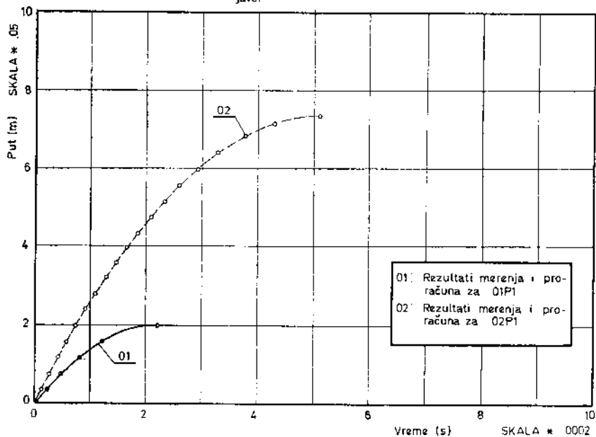
Sl. 7 Dubina penetracije zrna u funkciji vremena
