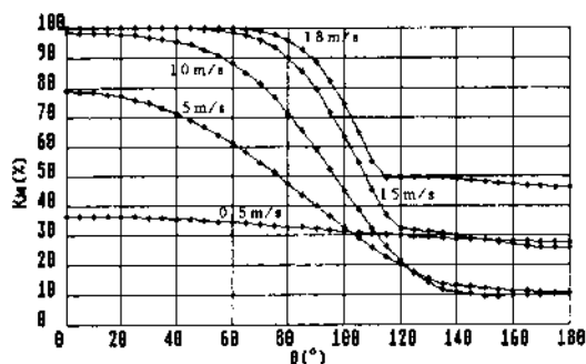
Sl. 16 Koeficijent smanjenja verovatnoće pogađanja u funkciji intenziteta i napadnog ugla vetra za kumulativnu municiju; Wr=0,5 do 18 \text{ m/s} ; Vt=25 \text{ km/h} ; tv=-30^\circ\text{C} ; X=2000 \text{ m}
