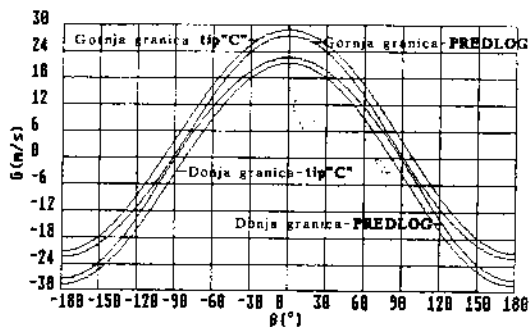
Sl. 22 Predložene maksimalne granice dozvoljenih odstupanja kod merenja intenziteta bočnog vetra u odnosu na granice, date za meteosenzor tipa »C«; W_r=25\text{ m/s} ; t_v=-30^{\circ}\text{C}
