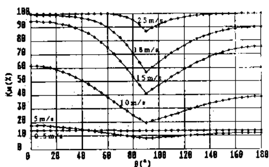
Sl. 20 Koeficijent smanjenja verovatnoće pogađanja u funkciji intenziteta i napadnog ugla vetra za kumulativnu municiju, kada se tenk kreće; Vt=0 \text{ km/h} ; Wr=0,5 do 25 \text{ m/s} ; tv=-30^\circ\text{C} ; X=2000 \text{ m}
