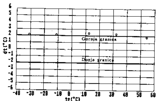
Sl. 12 Rezultati tačnosti merenja temperature meteosenzorom. W_r=3 \text{ m/s} ; p_v=1000 \text{ mbar}
