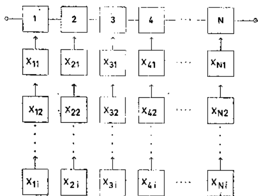
Sl. 1 Model TMS sa serijskom vezom sastavnih dijelova i rezervnim dijelovima u »hladnoj rezervi«
