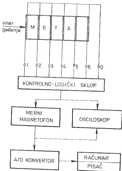
Sl. 2 Šema registracije i obrade signala
