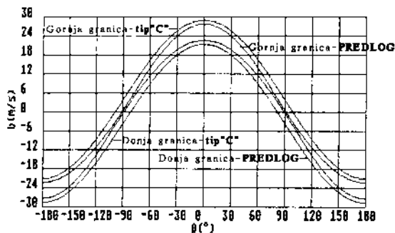
Sl. 21 Predložene maksimalne granice dozvoljenih odstupanja pri merenju intenziteta bočnog vetra u odnosu na granice date za meteosenzor tipa »C«; W_r=25\text{ m/s} ; t_v=15,9^{\circ}\text{C}
