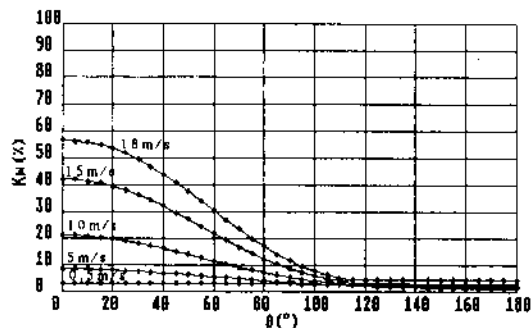
Sl. 18 Koeficijent smanjenja verovatnoće pogađanja u funkciji intenziteta i napadnog ugla vetra za trenutno-fugasnu municiju; Wr=0,5 do 18 \text{ m/s} ; Vt=25 \text{ km/h} ; tv=-30^\circ\text{C} ; X=2000 \text{ m}
