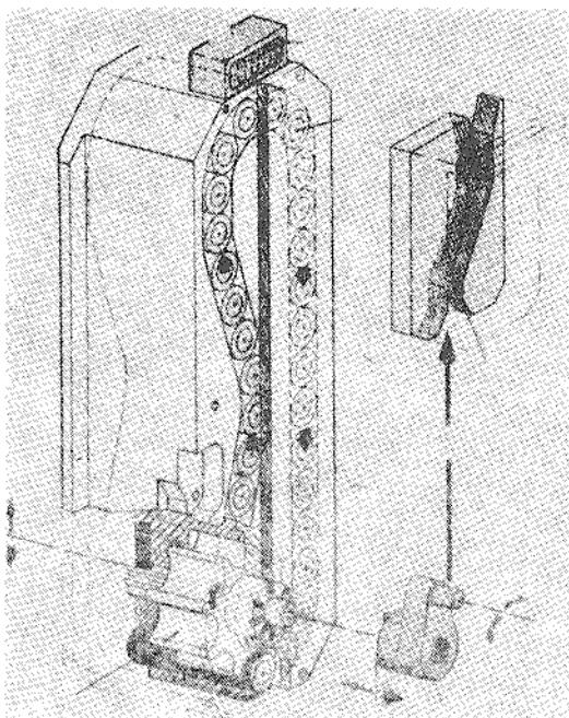
Poređenje zapremina ležišta metka topova sa cevima dužine 39 i 52 kalibra
