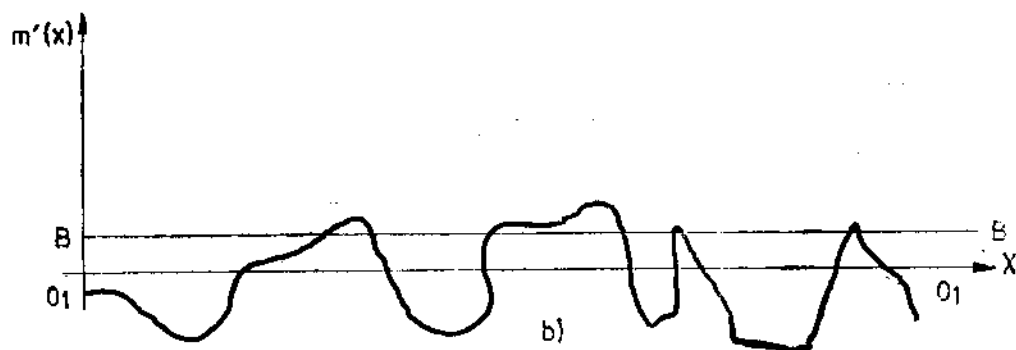
Sl. 4 Centriranje slučajne funkcije
