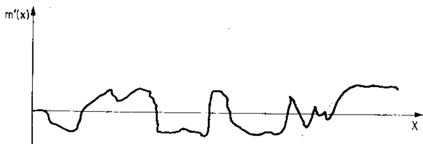
Sl. 1 Grafički prikaz slučajne funkcije
