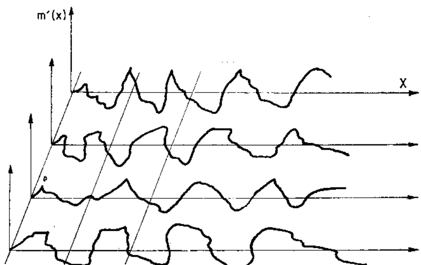
Sl. 2 Grafički prikaz skupa realizacija
