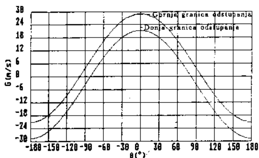
Sl. 5 Gornja i donja granica dozvoljenih maksimalnih odstupanja merenih vrednosti bočnog vetra meteosenzorom u funkciji napadnog ugla vetra
