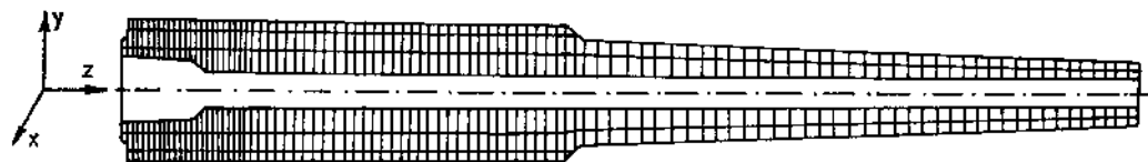
Sl. 2 Deo cevi podeljen na konačne elemente oblika pravougaoika, trapeza i trougla
