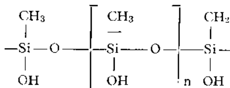
polimetilsiloksan
