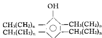
tetraparafin-fenol
