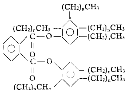
di(tetraparafin-fenol)ftalat
