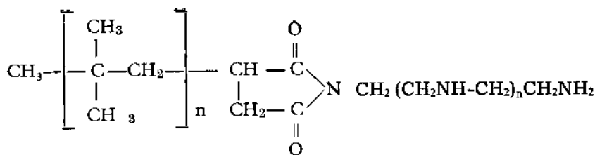
monosukcinimid
