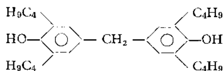
metilen-4,4-bis-(2,6-terc-butylfenol)
