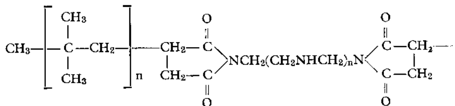
monosukcinimid
