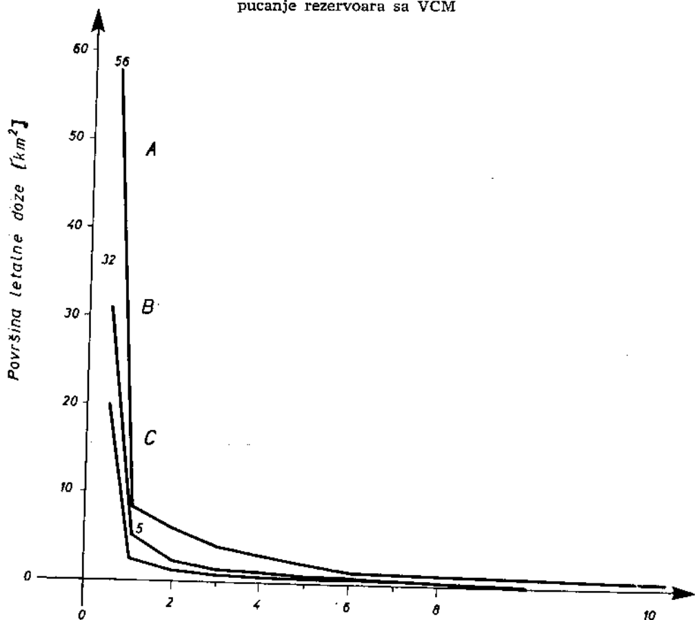
Sl. 3 Površina letalnih doza VCM: A — Pri istakanju 100%; B — Pri istakanju 50%; C — Pri istakanju 30%
