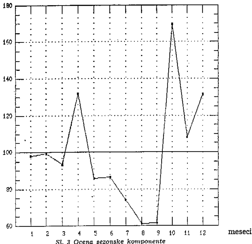
Sl. 3 Ocena sezonske komponente
