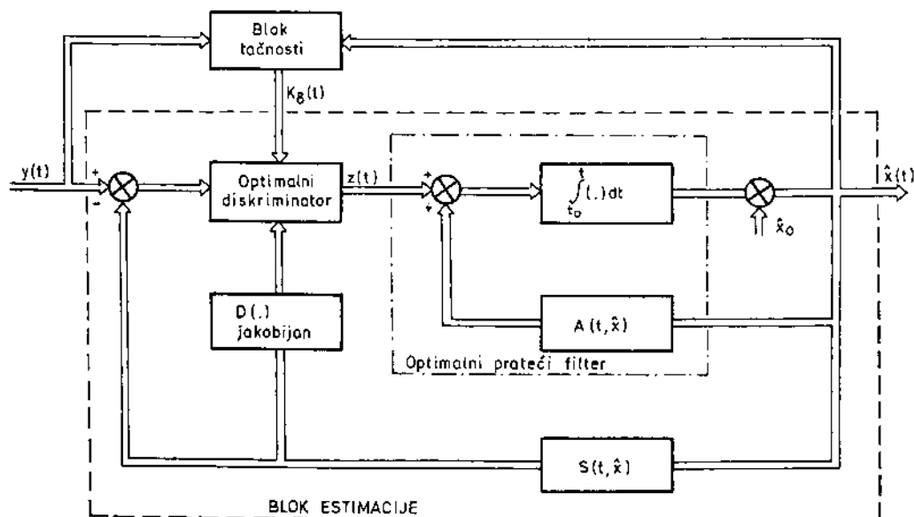
Sl. 3 Uopštena strukturna šema optimalne delinearne filtracije
