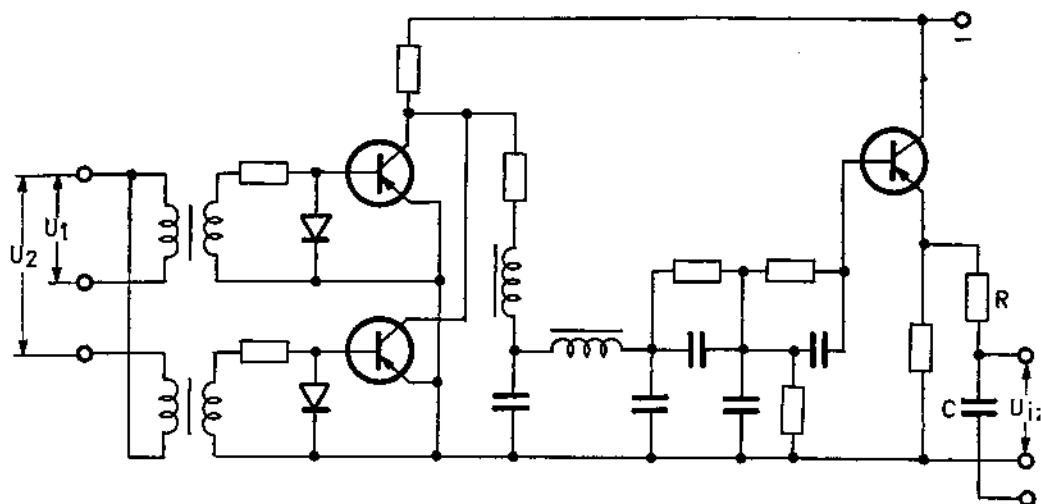
Sl. 7 Principijelna shema pretvarača ugla \theta u napon
