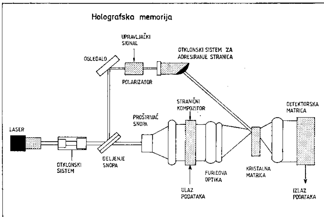
Sl. 14 Holografaska memorija
