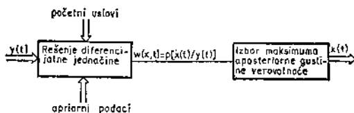
Sl. 2 Strukturna šema optimalne nelinearne filtracije sa opštim algoritmom
