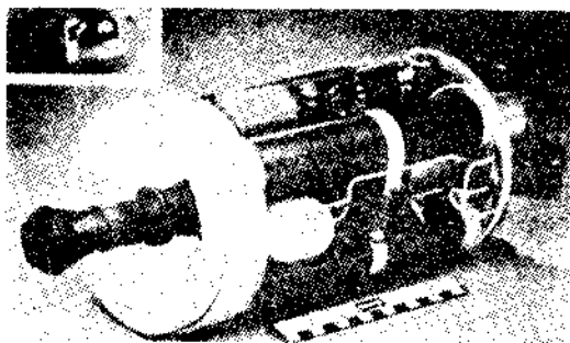
Maketa projektila LEAP sa minijturnim raketnim motorom
