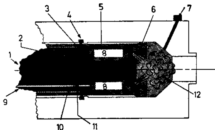
Sl. 2 Sematski presek i princip rada topa sa tečnim pogonskim punjenjem i regenerativnim ubrizgavanjem, koji ima sistem zadnjaka sa prstenastim linijskim klipom za ubrizgavanje;
