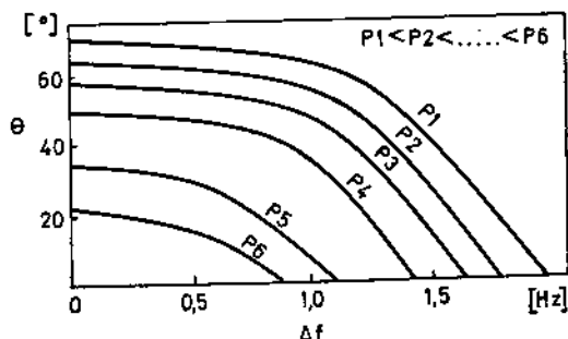
Sl. 4 Zavisnost ugla \theta od frekvencije \Delta f (parametar snaga sistema)
