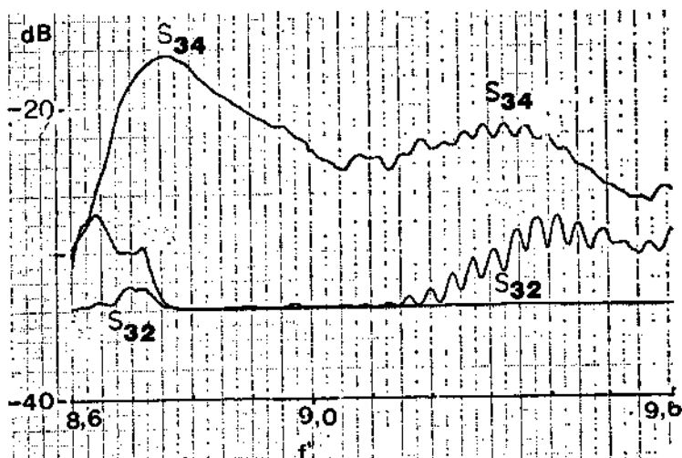
Sl. 4 Frekvencijska zavisnost sprege između sektora 3—4 i 3—2 antene sa sl. 1. S_{34} , S_{32} su apsolutne vrijednosti koeficijenta matrice raspršenja. Razmaci sektora antene su bili: A = 10,83 mm, B = 3,36 mm.
