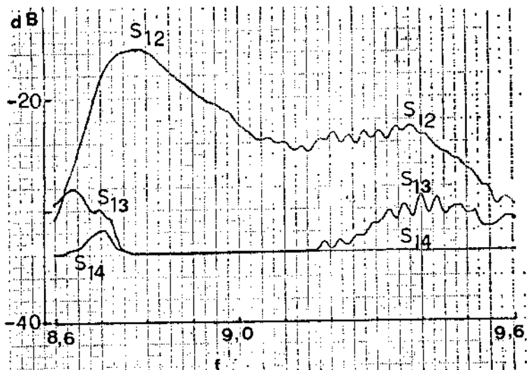
Sl. 3 Frekvencijska zavisnost sprege između sektora 1—2, 1—3, 1—4 antene sa sl. 1. S_{12} , S_{13} , S_{14} su apsolutne vrijednosti koeficijenta matrice raspršenja. Razmaci sektora antene su bili: A = 10,83 mm, B = 3,36 mm.
