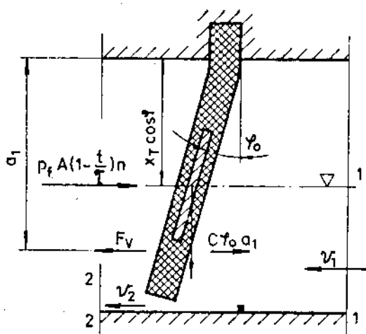
Sl. 2 Sema opterećenja membrane hidrauličkog protivudarnog ventila
