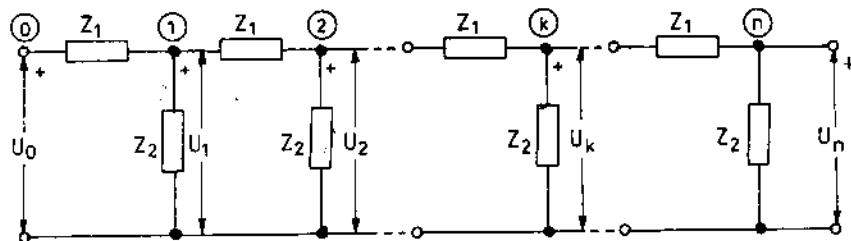
Sl. 1 Homogena ljestvičasta mreža
