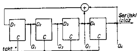
Sl. 2 — »Primjer generatora pseudoslučajnih binarnih brojeva«
