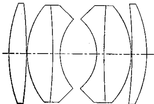
Sl. 7 — Optička šema kvazi simetričnog objektivâ
