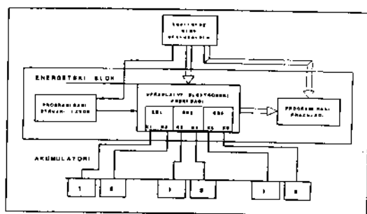
Sl. 5 — Blok šema sistema za ciklisanje Ni-Cd akumulatora
