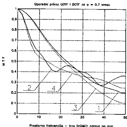
Sl. 10 — Uporedni prikaz GOTF i DOTF za ugao vidnog polja \omega = 0.7\omega_{\max}
