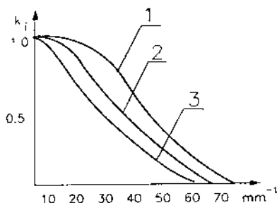
Sl. 3 — MTF objektivna za razne uglove upada u odnosu na optičku osu 1) za upadni ugao 0°; 2) za upadni ugao 10°; 3) za upadni ugao 30°
