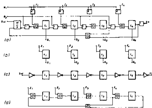
Sl. 7 — »Razne konfiguracije BILBO registra«
