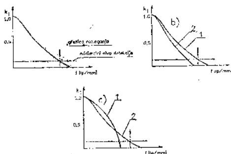
Sl. 2 — MTF lika u funkciji frekvencije testa a) za granični slučaj razlaganja i minimalni nivo detekcije; b) u slučaju jednostavnog, i c) u slučaju složenog određivanja kontrasta 1. i 2. optičkog sistema
