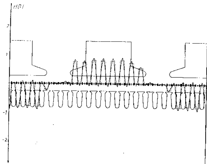
Sl. 4 — Raspodela magnetne indukcije na srednjoj liniji žleba rotora pri struji pobude I_f = 100\% I_{fn}
