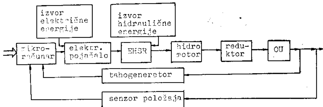
Sl. 1 — Principijelna shema elektrohidrauličnog sistema automatskog upravljanja
