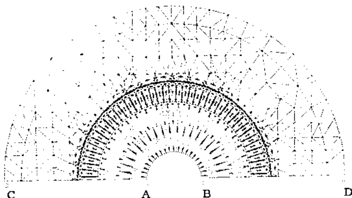
Sl. 2 — Mreža konačnih elemenata na jediničnom preseku sinhronog generatora
