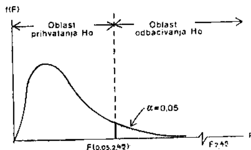
Sl. 4 — Kritična oblast za F_{2,45} \geq 1 , na nivou značajnosti \alpha=0,05 jedna od testiranih aritmetičkih sredi-
