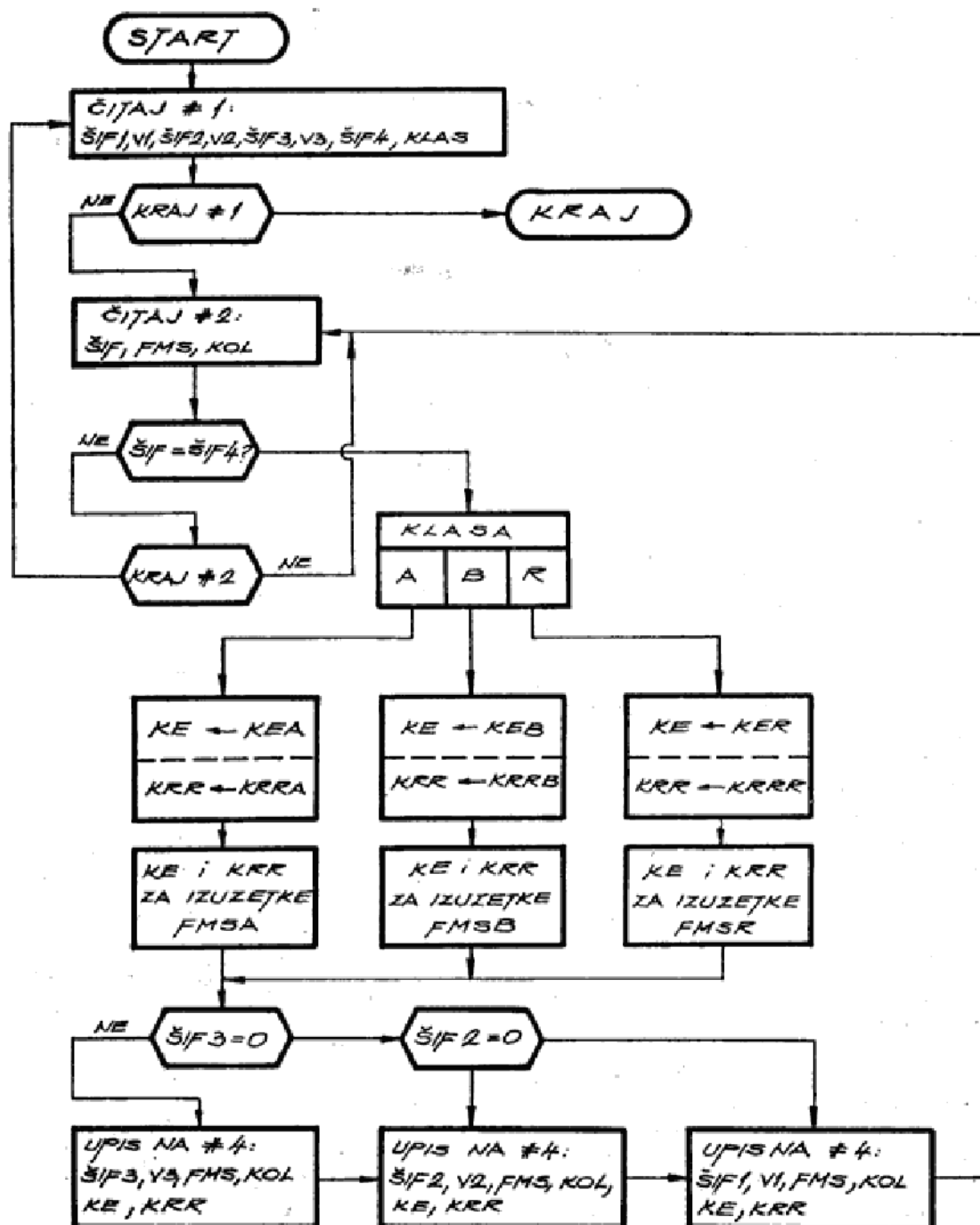
Sl. 3 — Blok dijagram programa KOEF
