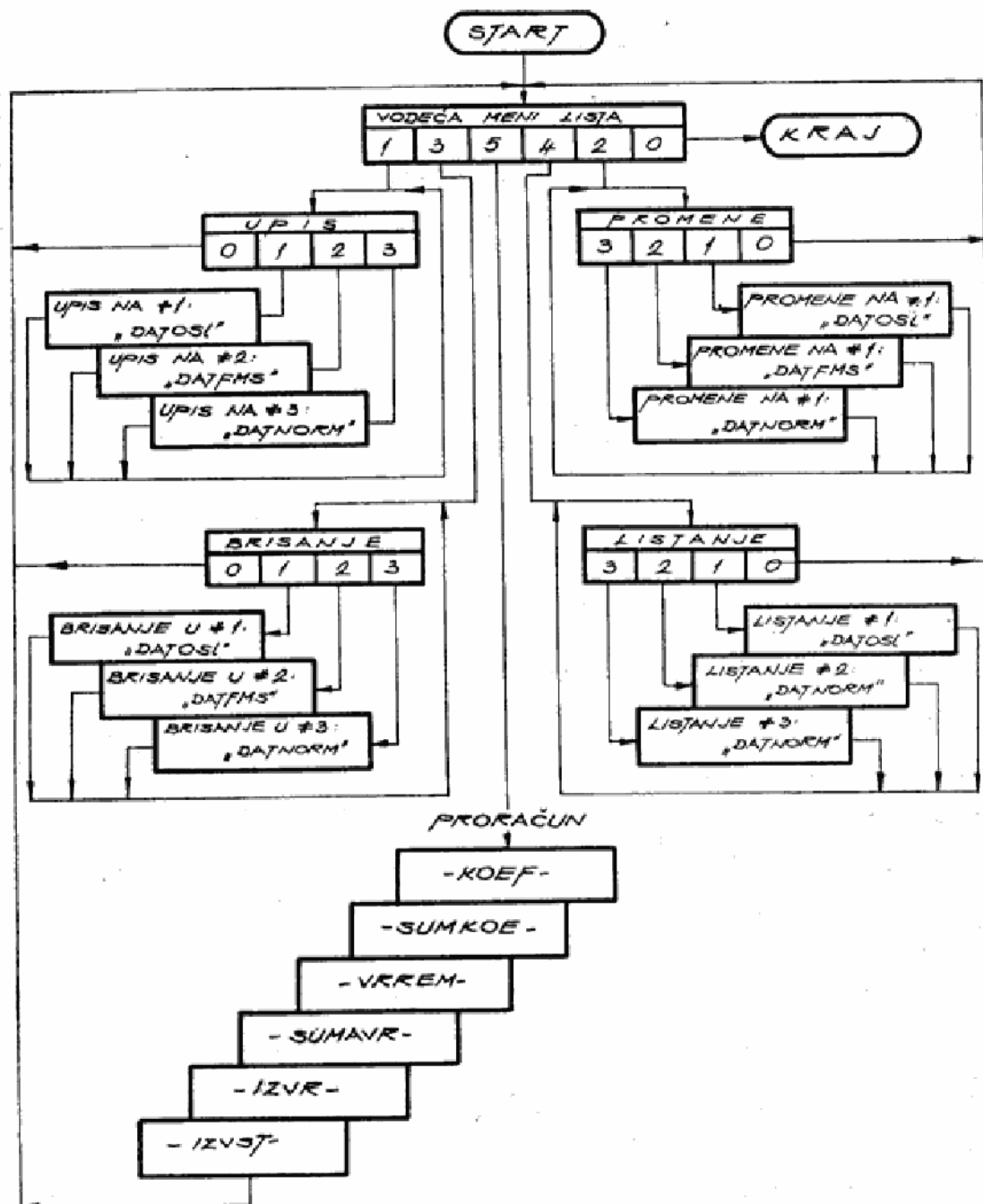
Sl. 1 — Blok dijagram programskog sistema
