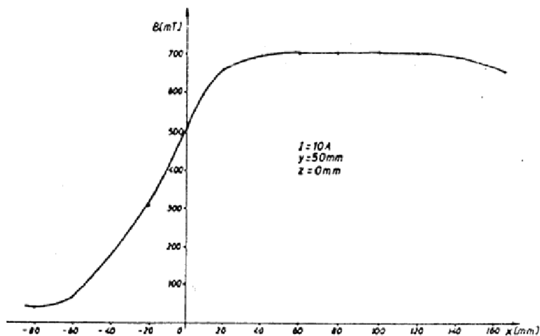
Sl. 15 — Raspodela magnetnog polja za struju od 10 A
