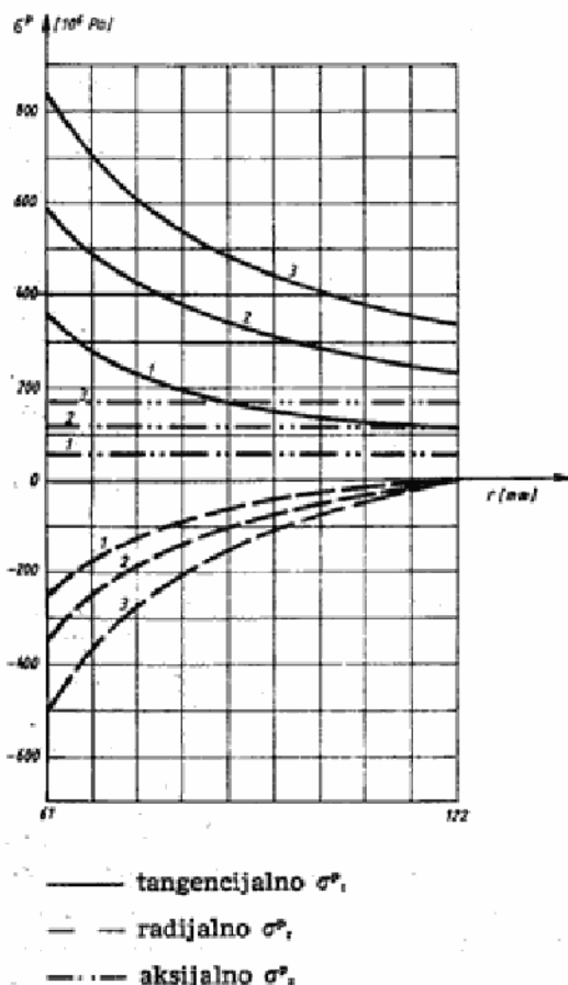
Sl. 3 — Naprezanje usled pritiska
