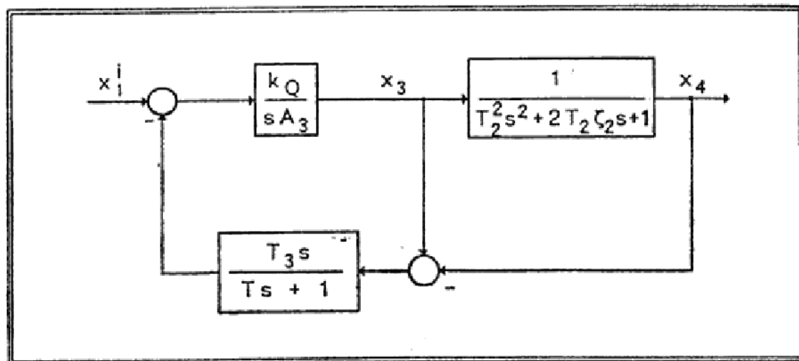
Sl. 4 — Transformirana strukturna shema
