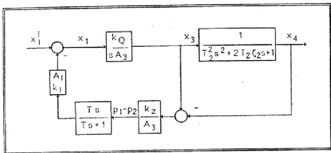
Sl. 3 — Transformirana strukturna shema servosistema
