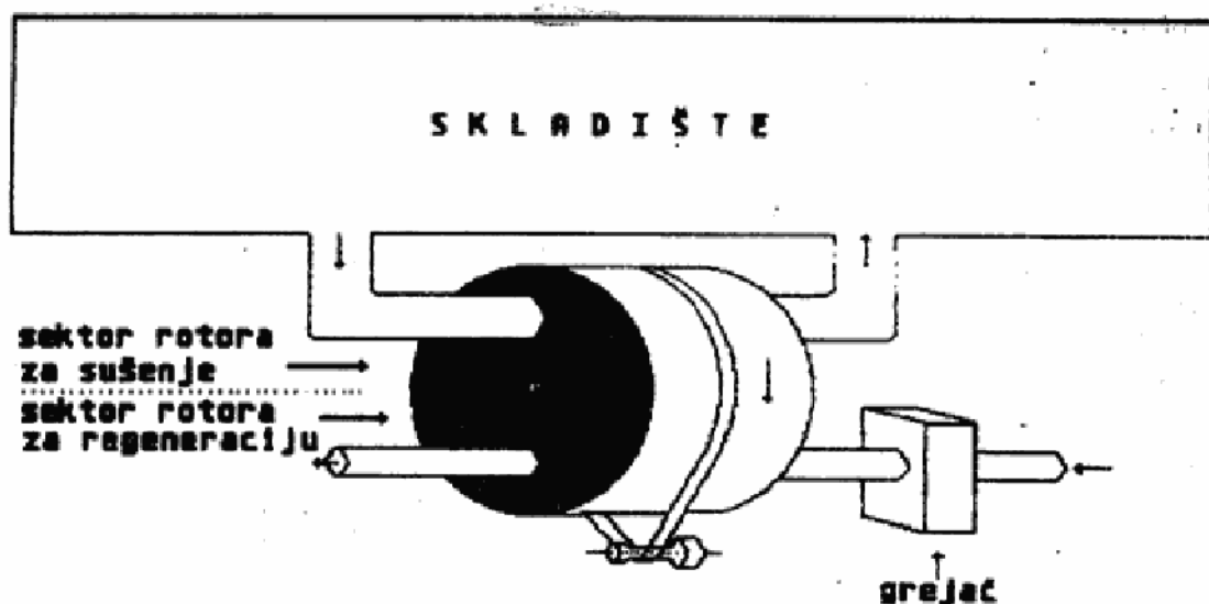
Sl. 3 — Šematski prikaz rada agregata za dinamičko odvlaživanje
