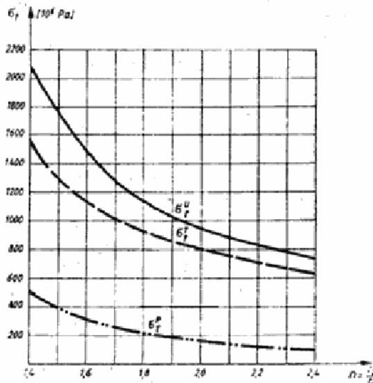
Sl. 2 — Tangencijalno naprezanje na radijusu r_1
