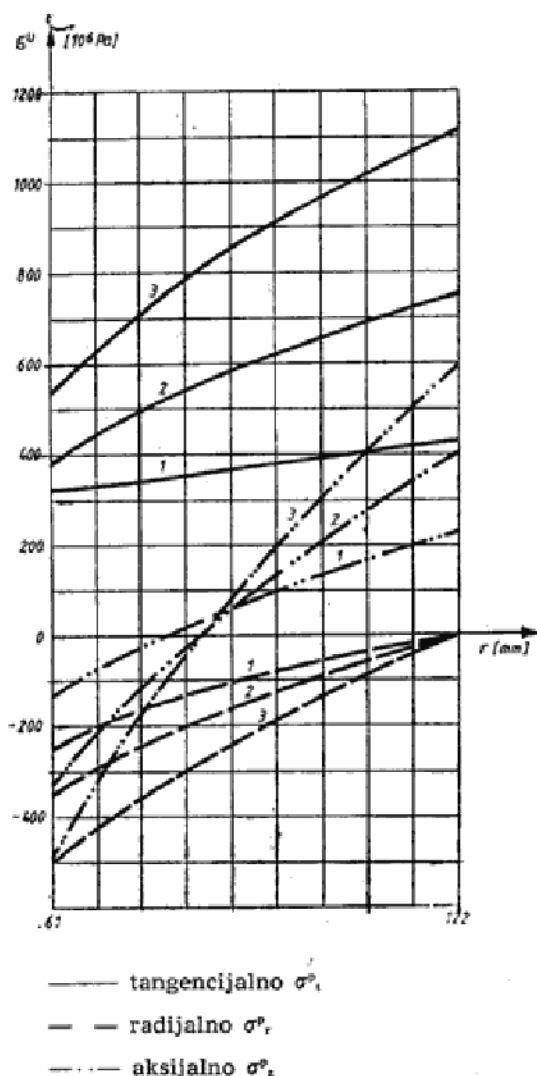
Sl. 5 — Ukupna naprezanja
