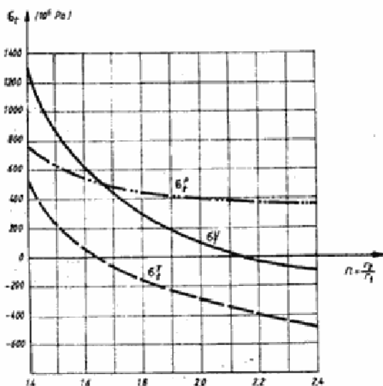
Sl. 1 — Tangencijalno naprezanje na radijusu r_1
