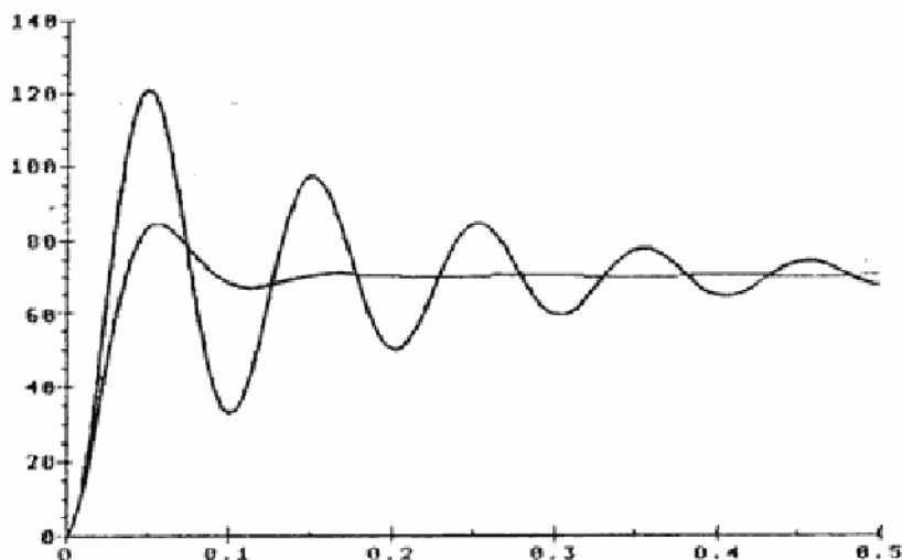
Sl. 5 — Vremenski odziv na jediničnu step-funkciju
