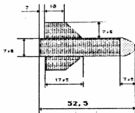
Sl. 5 — Dimenzije modela rakete
