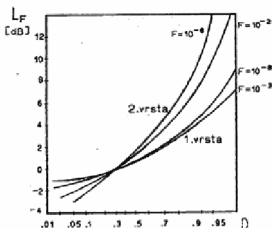
Sl. 4 — Zavisnost koefficijenta gubitaka od verovatnoće otkrivanja ciljeva ( D )
