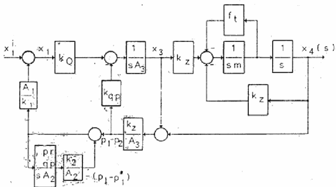
Sl. 2 — Detaljna strukturna shema servosistema
