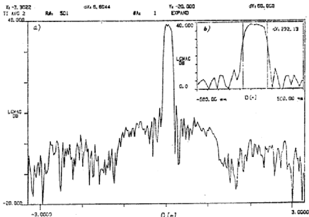
Sl. 4 — Distribucija »bleštećih« tačaka diska: a) u opsegu od 6,6 m, b) u opsegu od 1 m
