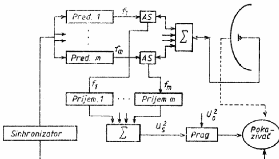
Sl. 2 — Blok shema frekventno-diverziti radarskog sistema [6]
