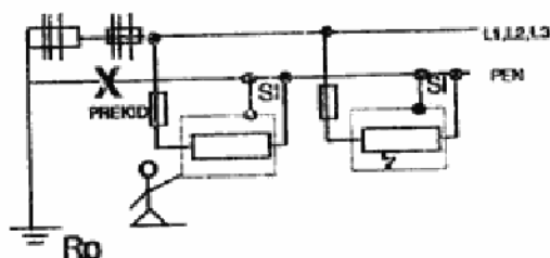
Sl. 10 — Prekid nulvoda — fazni napon na nulvodu
