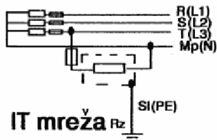
Sl. 1 — Tipovi mreža
