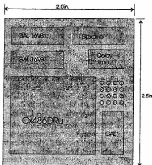
Sl. 2 — Cyrix-ov cip DKu 2 je direktna zamena (nožica na nožicu) za Intel 386DX/20. Glavni mikroprocesor je najveći kvadrat u donjem levom uglu. Ostale jedinice na pločici 2x2.5 inča su pomoćni čipovi
