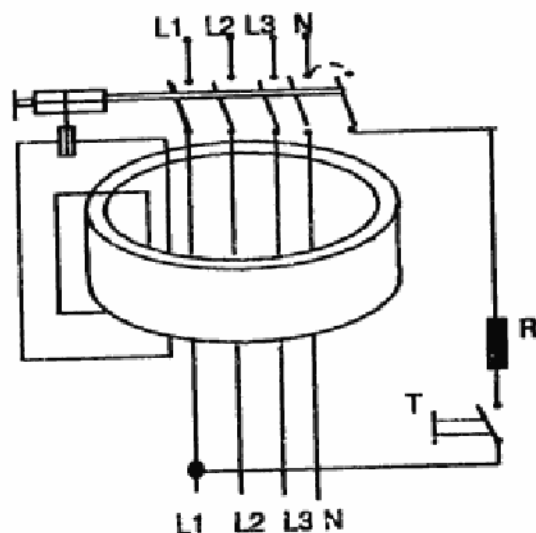
Sl. 5 — Strujna zaštitna sklopka (FI)
