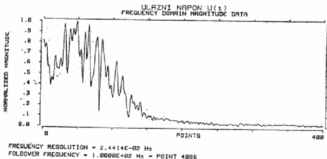
Sl. 4 — Frekventni spektar obojenog šuma
