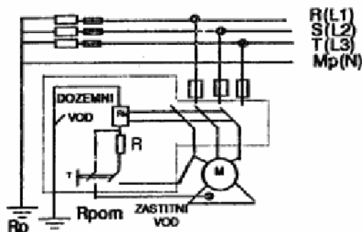
Sl. 9 — Naponska zaštitna sklopka (FN)
