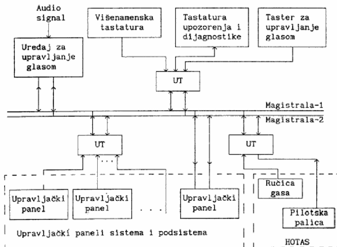
Sl. 5 — Arhitektura upravljačkog dela UPP-a
