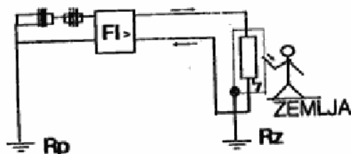
Sl. 6 — Princip delovanja FI sklopke
