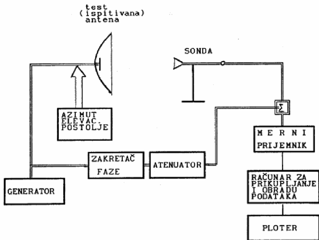
Sl. 7 — Merni sistem za merenje mikrotalasnog holograma
