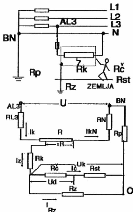
Sl. 2 — Uzemljeno pogonsko sredstvo sa naddomesnom shemom
