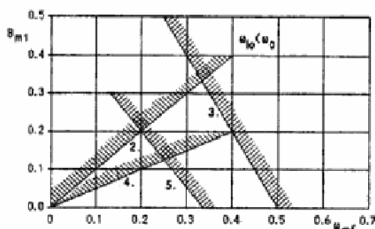
Slika 7 — Ukupni frekventni kriterijumi nastajanja IM produkata u mešaču kod kojega je \omega_{10} < \omega_0
