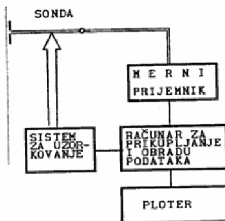
Sl. 5 — Merni sistem za merenje u bliskom polju
