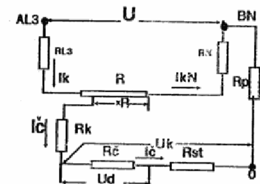
Sl. 15 — Neuzemljeno pogonsko sredstvo sa nadomesnom shemom
