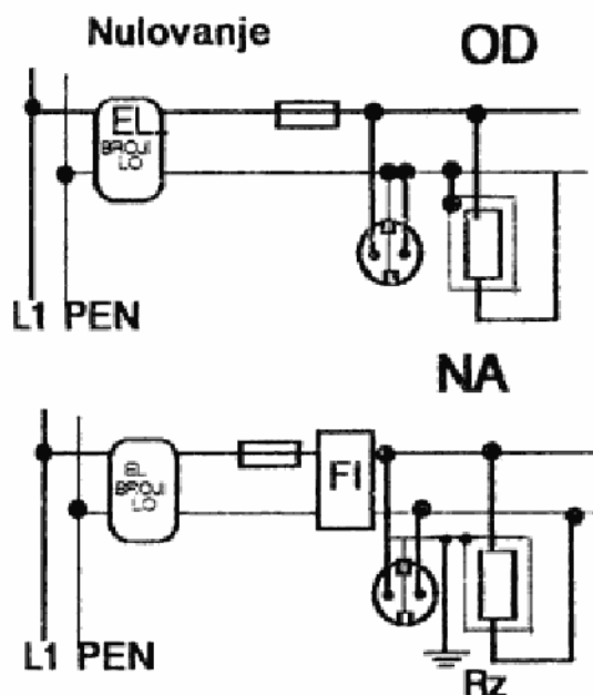
Sl. 7 — Upotreba FI sklopke kod TN mreže
