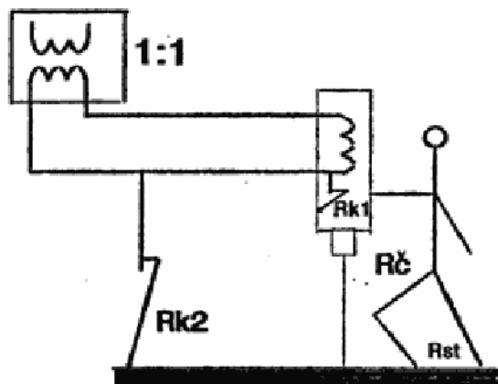
Sl. 16 — Zaštitno odeljivanje
