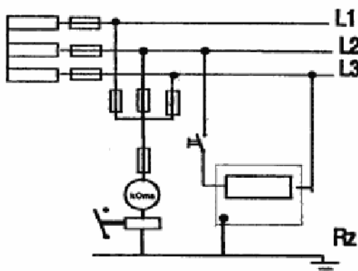
Sl. 14 — Kontrolnik izolacije
