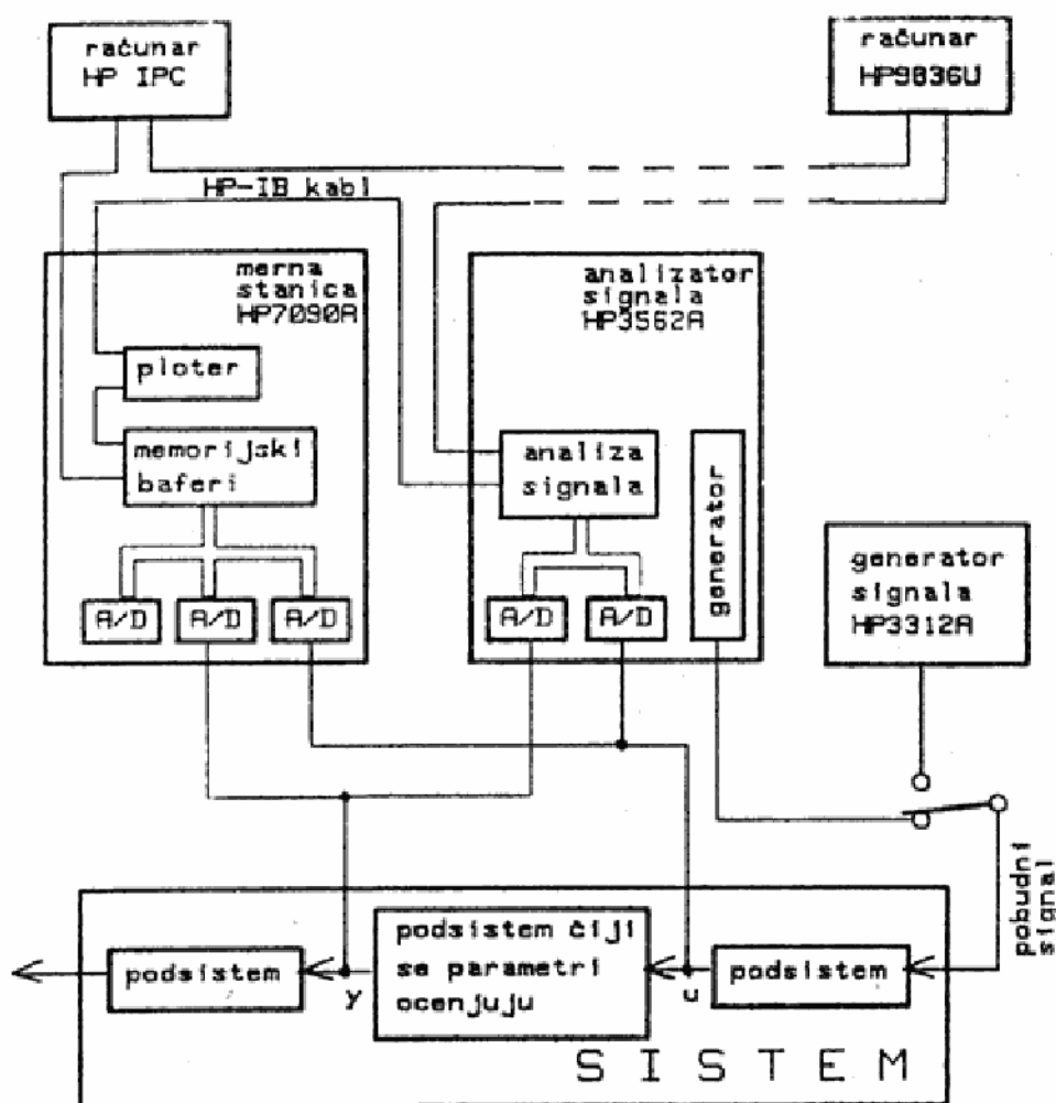
Sl. 1 — Merni sistem
