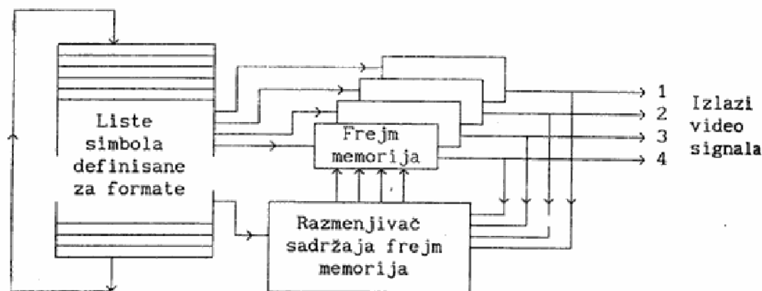
Sl. 6 — Softversko preključivanje video-signala
