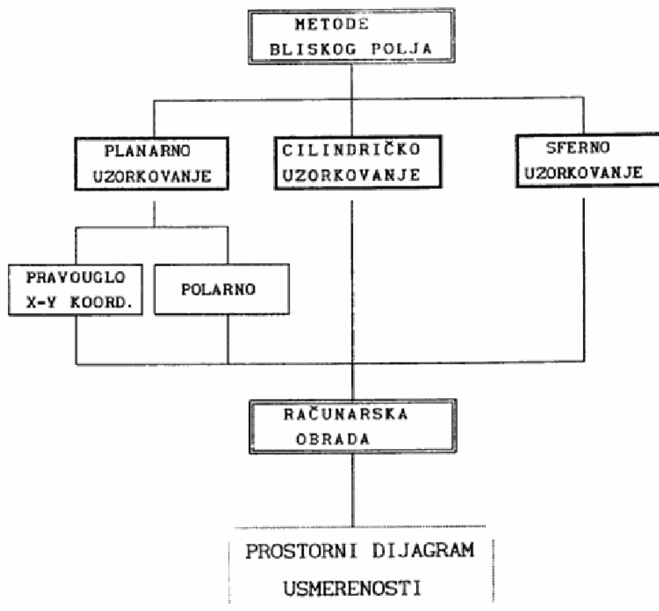
Sl. 4 — Vrste mernih metoda bliskog polja
