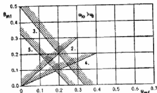
Slika 6 — Ukupni frekventni kriterijumi nastajanja IM produkata u mešaču kod kojega je \omega_{10} > \omega_0
