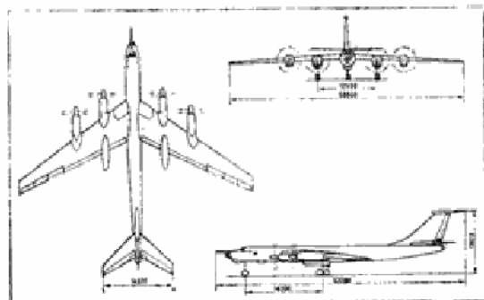
Sl. 1 — Protivpodmornički avion Tu-142M
