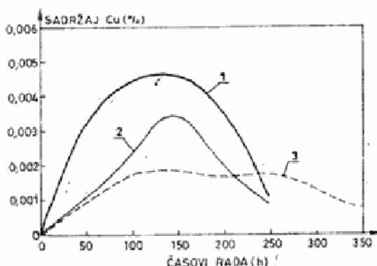
Sl. 16 — Sadržaj Cu u motornom ulju 1 — motor DM33/T sa RME, 2 — motor M33/T sa RME, 3 — motor M33/T sa D2
