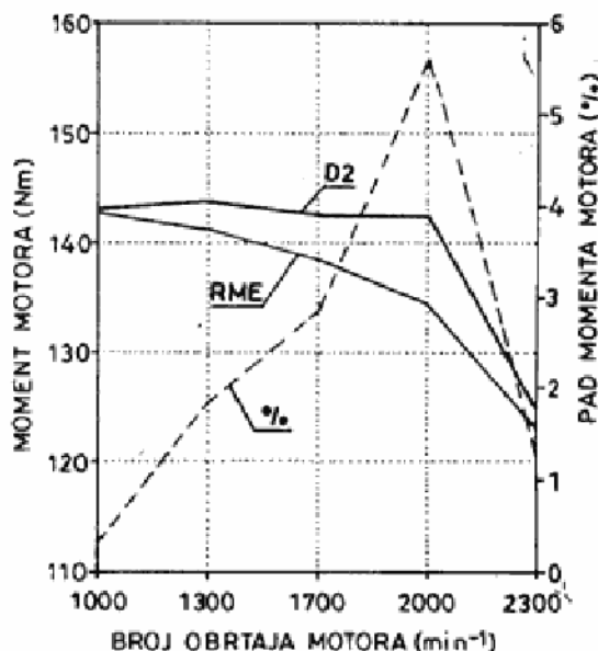
Sli. 8 — Uporedni dijagram momenta motora M33
