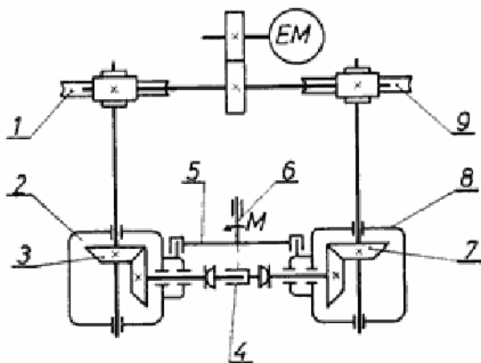
Sl. 6 — Uređaj sa dva obrtna kućišta
