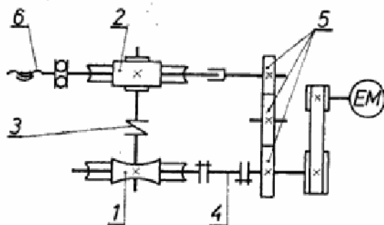
Sl. 8 — Uređaj za ispitivanje globoidnih pužnih prenosnika
