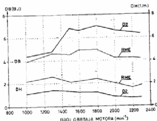
Sl. 19 — Emisija dima
