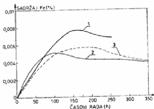
Sl. 15 — Sadržaj Fe u motornom ulju 1 — motor DM33/T sa RME, 2 — motor M33/T sa RME, 3 — motor M33/T sa D2
