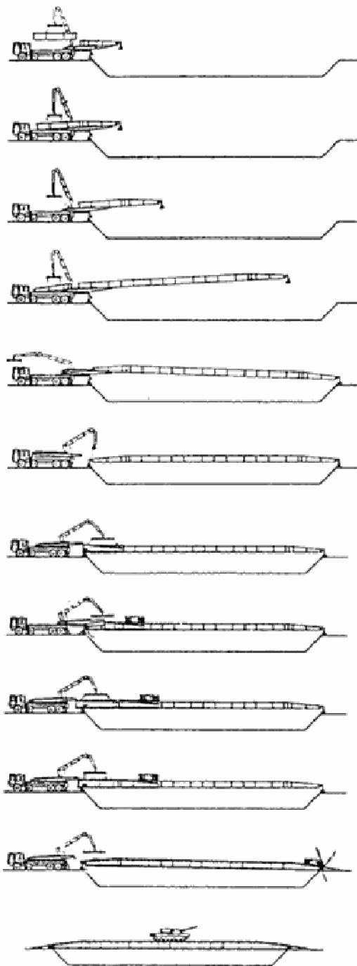
Sl. 1 — Redosled polaganja probnog mosta DoFB
