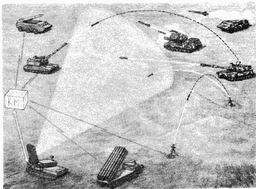
Sl. 2 — Princip rada izviđačkog sistema ZOOPARK-1
