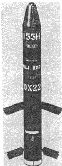
Sl. 1 — Vodeni artiljerijski projektil 155 mm M-712
