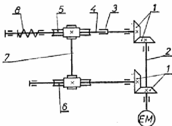
Sl. 7 — Uređaj sa opterećivanjem aksijalnim pomeranjem puža
