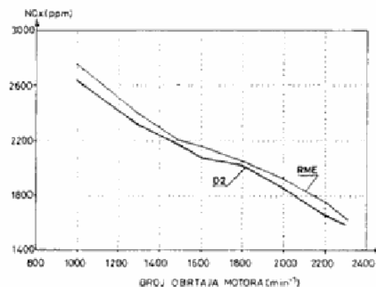
Sl. 20 — Emisija azotovih oksida NO_x
