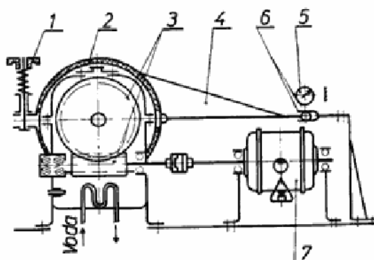
Sl. 1 — Uređaj sa papučastom kočnicom
