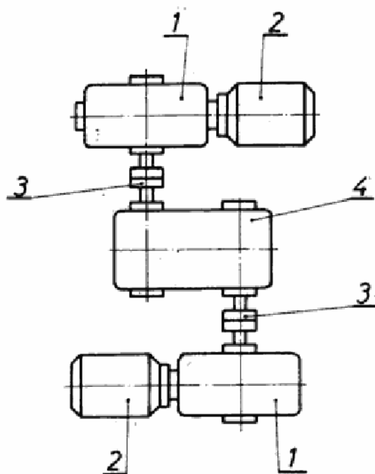
Sl. 2 — uređaj sa kočionim generatorom
