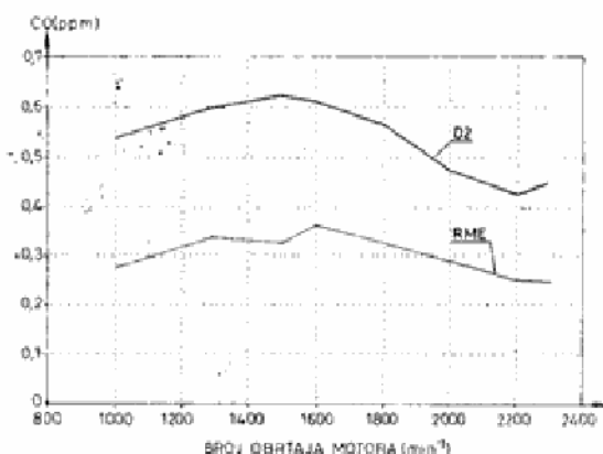
Sl. 22 — Emisija ugljenmonoksida CO
