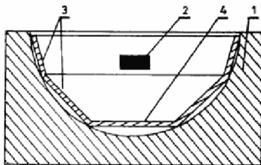
Sl. 5 — Oblikovanje sfernih kupola preoblikovanjem u segmente
