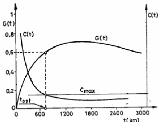
Sl. 3 — Kompromisni izbor najpovoljnijeg rešenja (trade-off)
