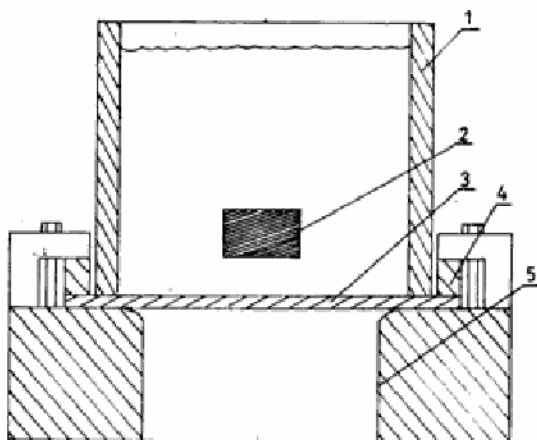
Sl. 2 — Eksplozivno slobodno oblikovanje u otvorenoj matrici
