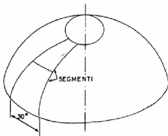
Sl. 6 — Sferna kupola sastavljena iz segmenata
