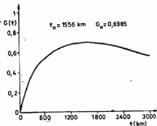
Sl. 1 — Izlazna operaciona karakteristika modela MAXGOT
