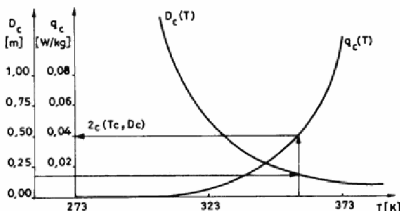
Sl. 1 — Izlazni dokument sa mikrokalorimetra — grafička zavisnost D_c(T) i q_c(T)
