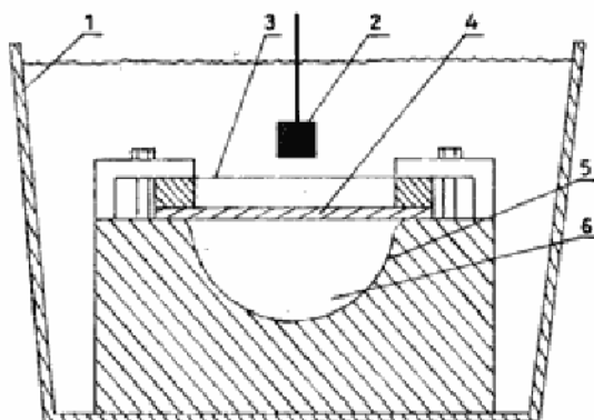
Sl. 1 — Oblikovanje eksplozijom u zatvorenoj matrici
