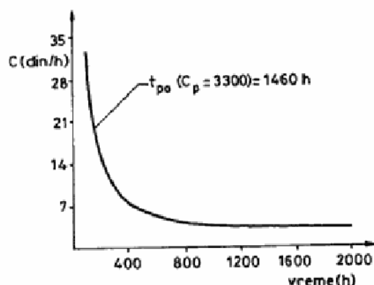
Sl. 2 — Izlazna operaciona karakteristika modela MINTRO
