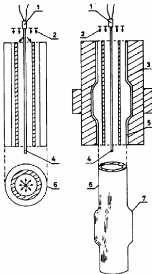
Sl. 7 — Oblikovanje cevastih komponenti eksplozijom
