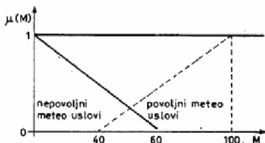
Sli. 3 — Funkcije pripadnosti fuzzy skupova »nepovoljni meteorološki uslovi« i »povoljni meteorološki uslovi«
