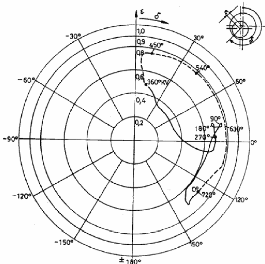
Sl. 6 — Dinamička putanja rukavca kolenastog vratila
