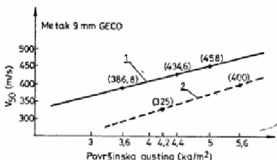
Sl. 5 — Poređenje balističke otpornosti Kevlara
