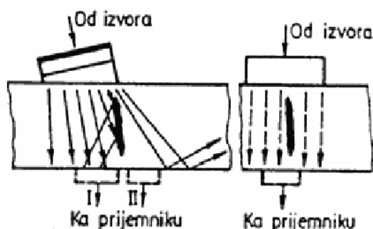
SL. 4 — Šema metoda senke ultrazvučne defektoskopije
