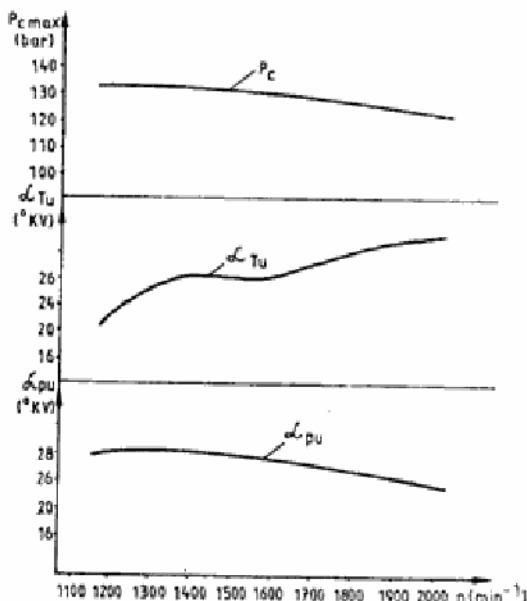
Sl. 2 — Promena maksimalnog pritiska sagorevanja p_{\max} , ugla početka \alpha_n i trajanja ubrizgavanja \alpha_n u zavisnosti od brzine obrtanja kolenastog vratila
