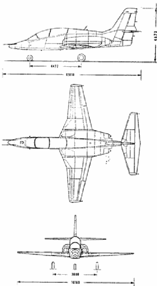
Sl. 2 — Dimenzije aviona MiG-AT
