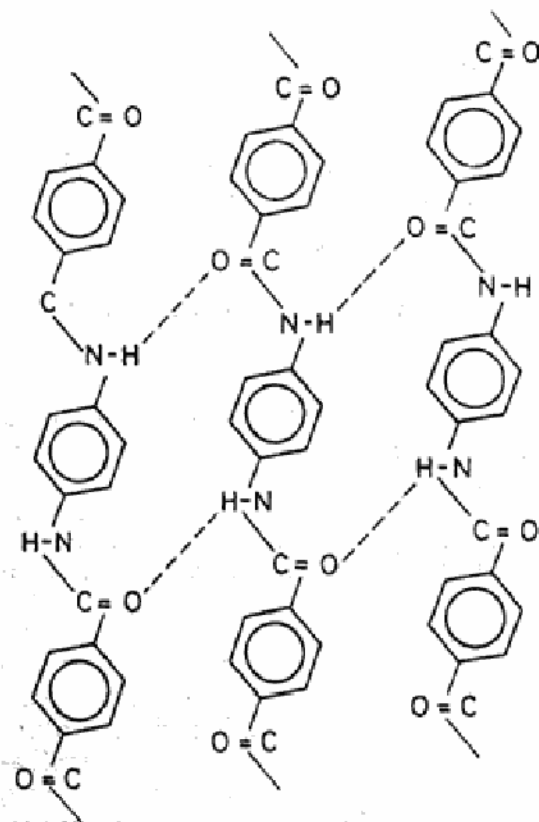
Sl. 1 — Hemijska struktura vlakana Kevlara
