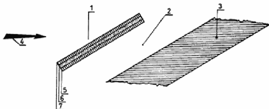
Sl. 4 — Šema ukošenog razdvojenog »sendvič« oklopa
