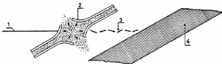
Sl. 5 — Sema uzajamnog dejstva kumulativnog mlaza i »sendviča« sa inertnim međuslojem
