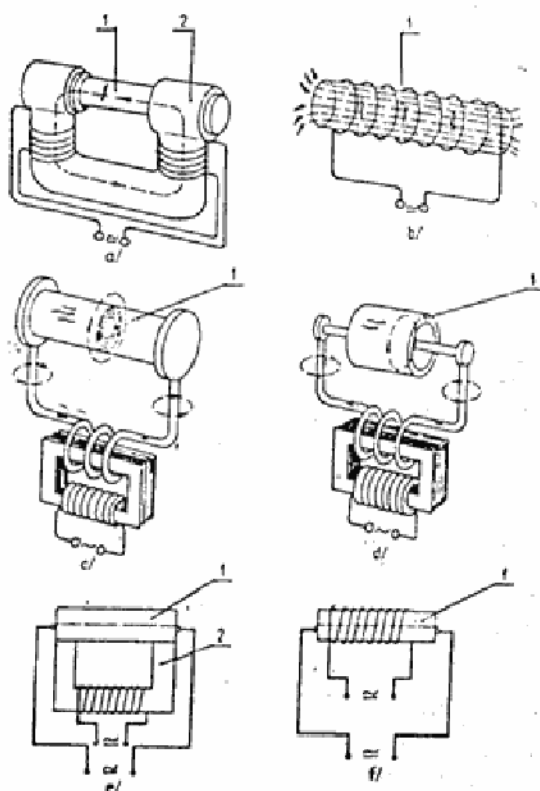
Sl. 1 — Šema namagnetisavanja elemenata a, b — polarno, c, d — cirkulaciono, e, f — kombinovano, 1 — ispitivani elemenat koji se magnetise, 2 — elektromagnet
