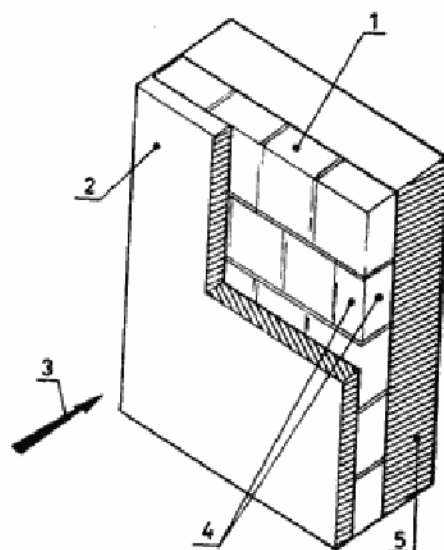
Sl. 1 — Šema oklopa sa keramičkim pločama
