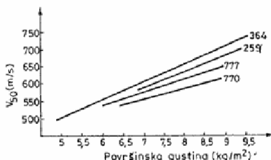
Sl. 4 — Balistička otpornost različitih prediva Kevlara
