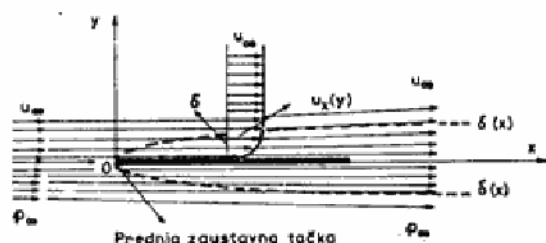
Sl. 1 — Karakteristike graničnog sloja oko ravne ploče
