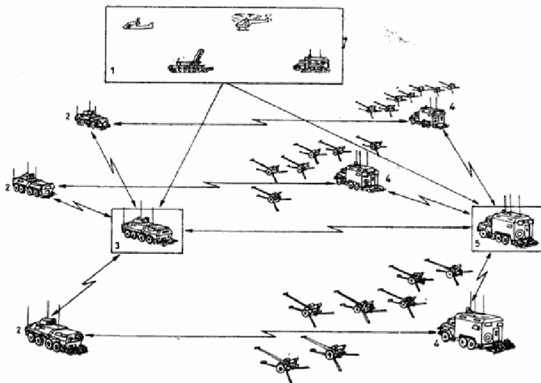
Sl. 1 — Sema automatskog sistema za upravljanje vatrom
