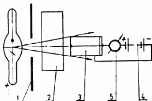
Sl. 3 — Jonizacioni metod defektoskopije
