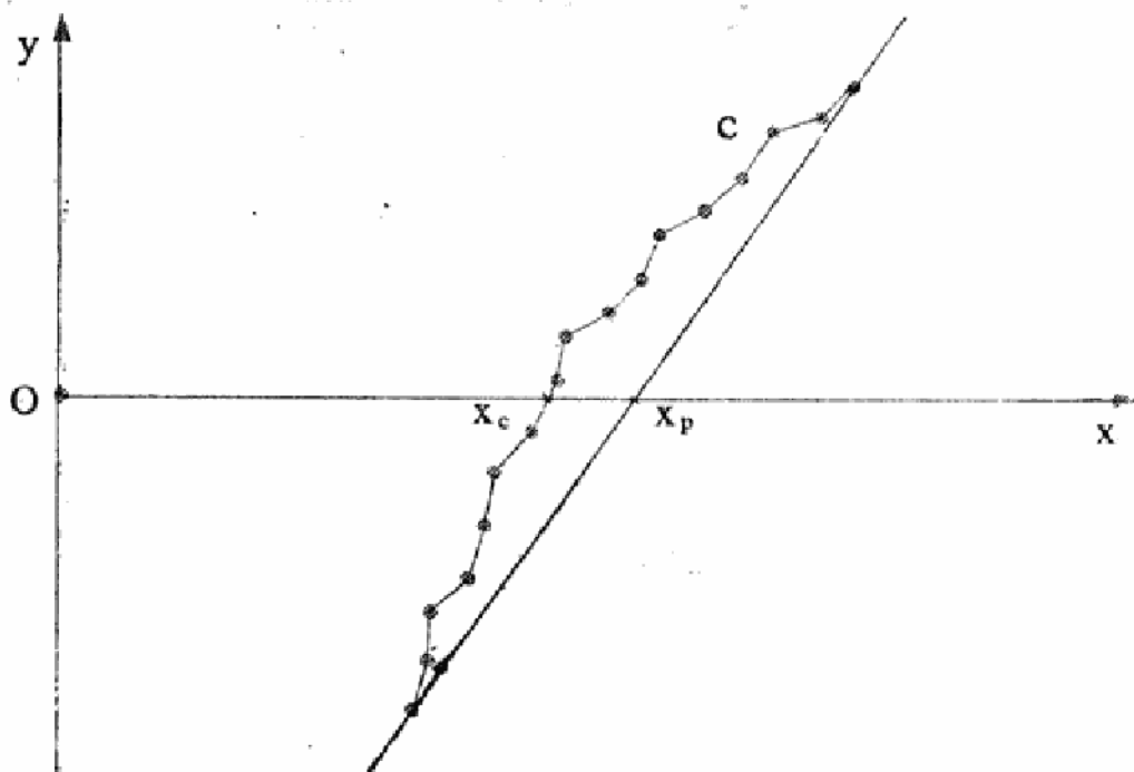
Sl. 1 — Henrijeva kriva
