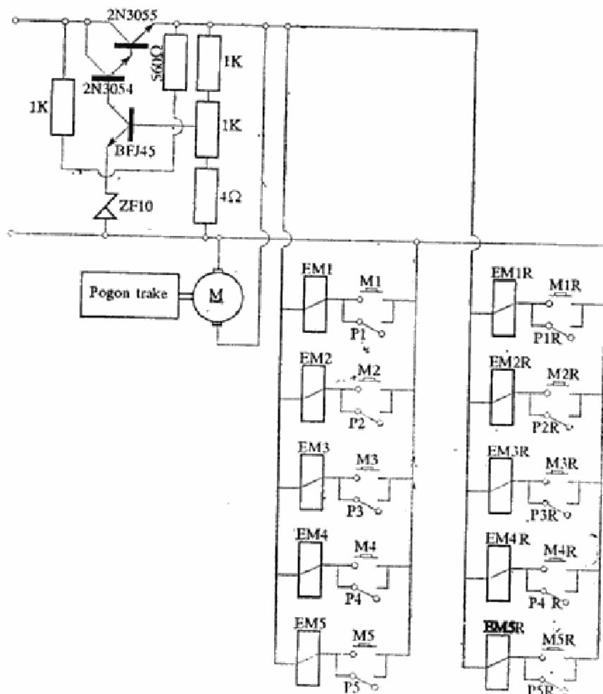
Sl. 1 — Električna šema uređaja za zapisivanje podataka:
