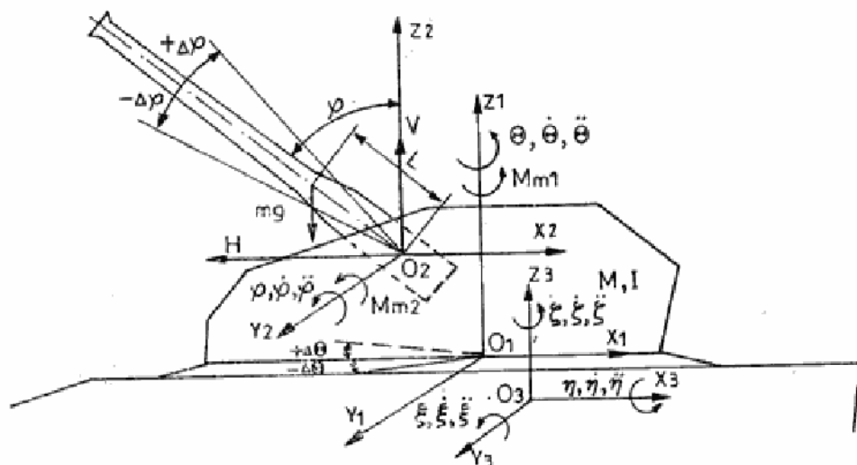
Sl. 2 — Kinematska struktura objekta upravljanja
