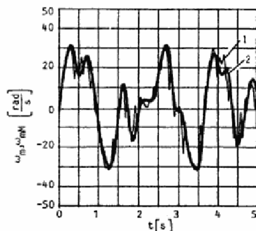
Sl. 8 — Odziv elektromotora
