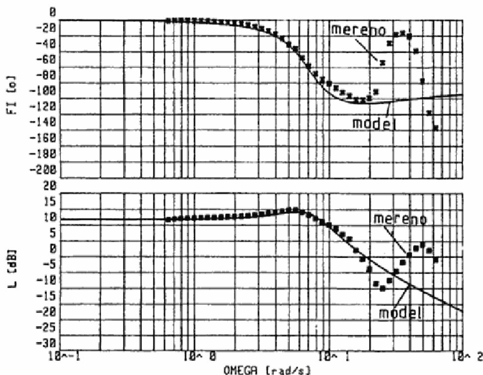
Sl. 5 — Frekventna karakteristika električnog servosistema
