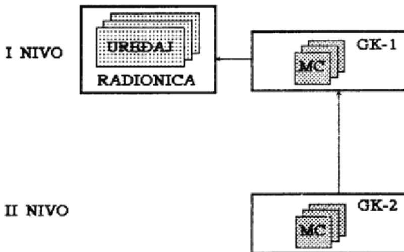
Sl. 2 — Korektivno održavanje elektronskog uređaja neopravljivim MC
