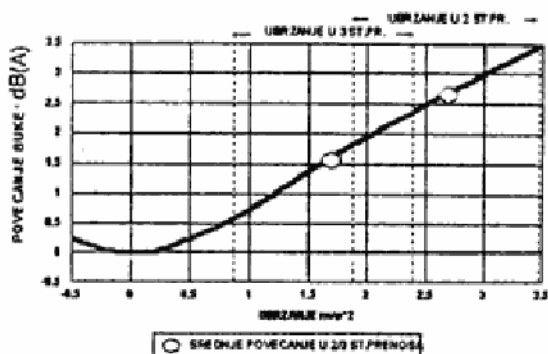
Sl. 11 — Uticaj ubrzanja vozila na buku pneumatika
