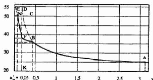
Sl. 8 — Zavisnost čvrstoće \delta_m spoja titan-čelik od relativne debljine mekog međusloja ( x )
