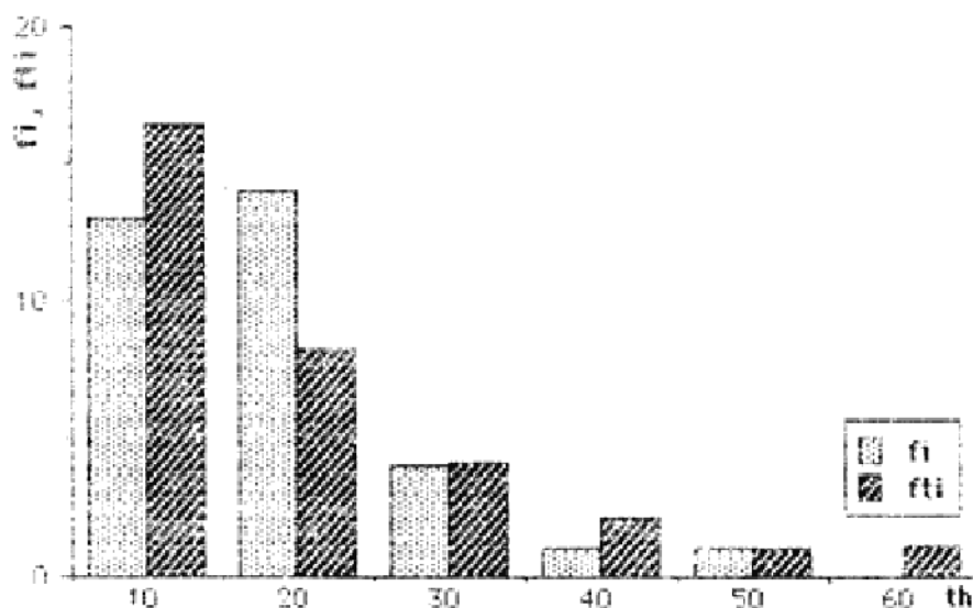
Sl. 6 — Histogram frekvencija — merno mesto br. 4, Lazarica
