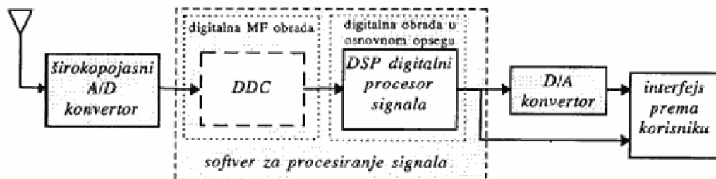
Sl. 2 — Struktura softverskog prijemnika
