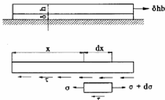
Sl. 3 — Uslovi ravnoteže elementa dx
