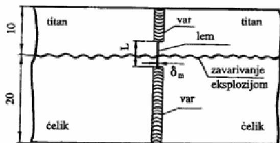
Sl. 5 — Šema sučeonog spajanja titana i čelika
