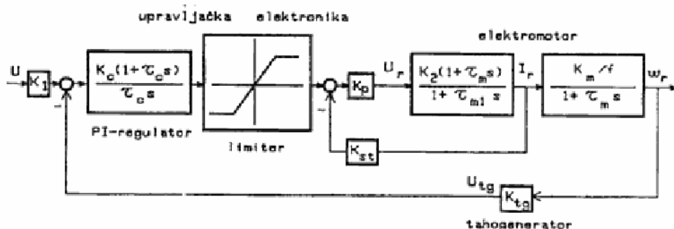
Sl. 2 — Blok-dijagram električnog servosistema
