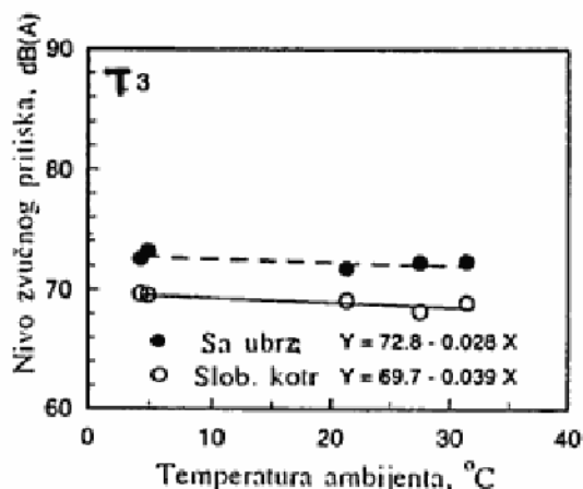
Sl. 4 — Zavisnost nivoa buke i temperature ambijenta za pneumatike lakih kamiona
