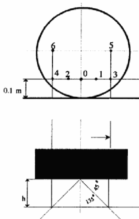
Sl. 2 — Položaj mikrofona pri merenju buke pneumatika:
