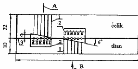
Sl. 6 — Šema određivanja temperature pri zavarivanju bimetalna titan-čelik:
