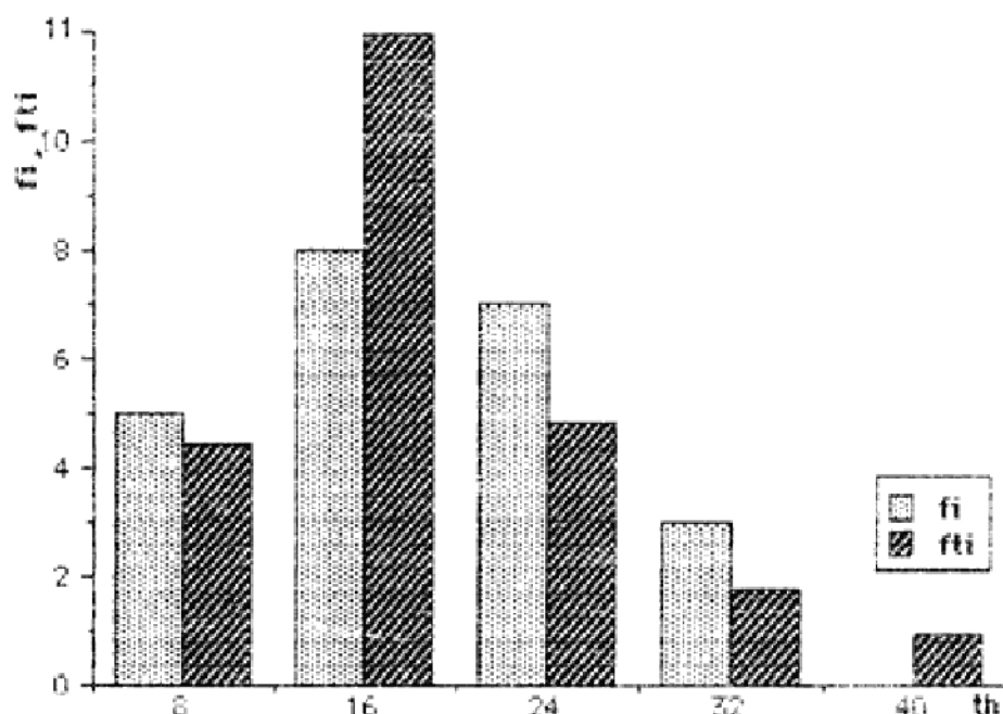
Sl. 4 — Histogram frekvencija — merno mesto br. 2, Počkovina
