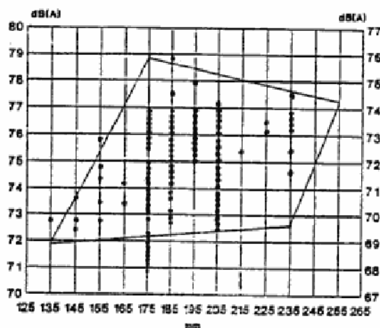
Sl. 13 — Buka 143 različitih tipa pneumatika u zavisnosti od uslova ispitivanja
