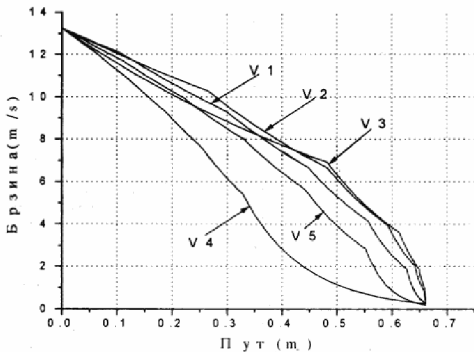
Sl. 3 — Zavisnost brzine od puta kočenja
