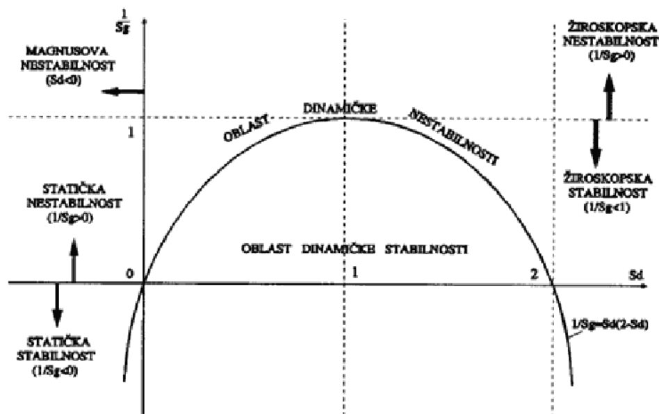
Sl. 1 — Granična kriva stabilnosti
