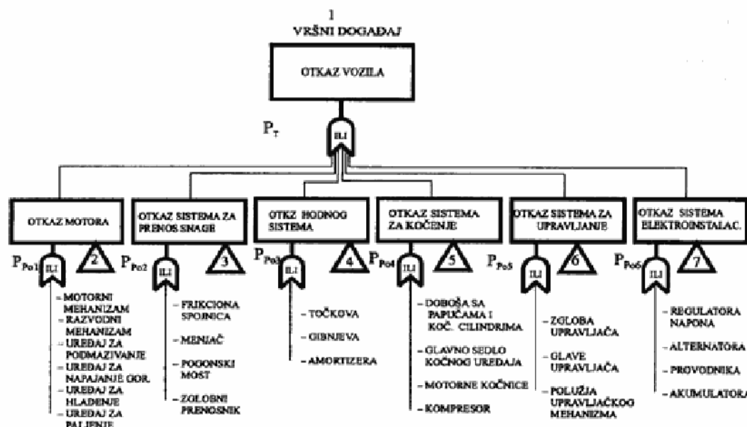
Sli. 1 — Struktura stabla otkaza za vršni događaj — otkaz vozila
