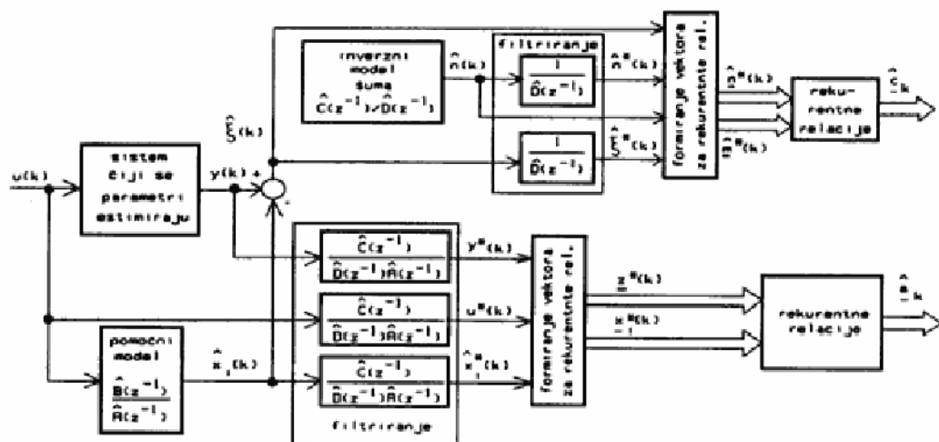
Sl. 1 — Metoda najveće verodostojnosti
