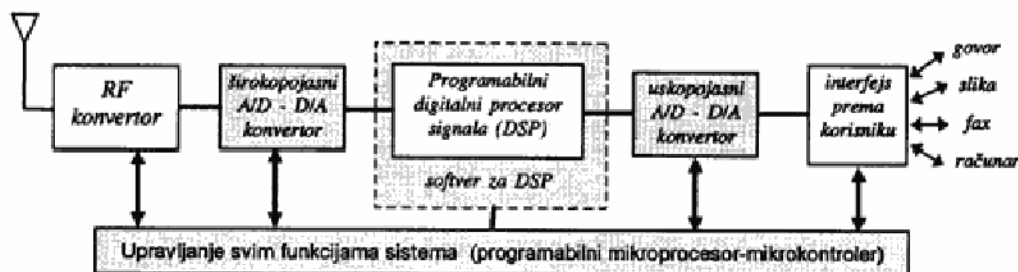
Sl. 1 — Blok-šema softverskog radija
