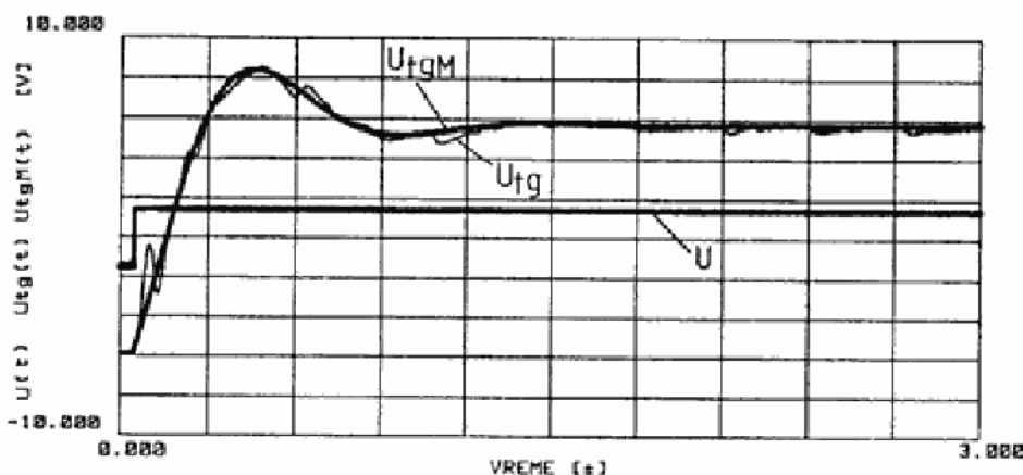
Sl. 6 — Odskočni odziv električnog servosistema
