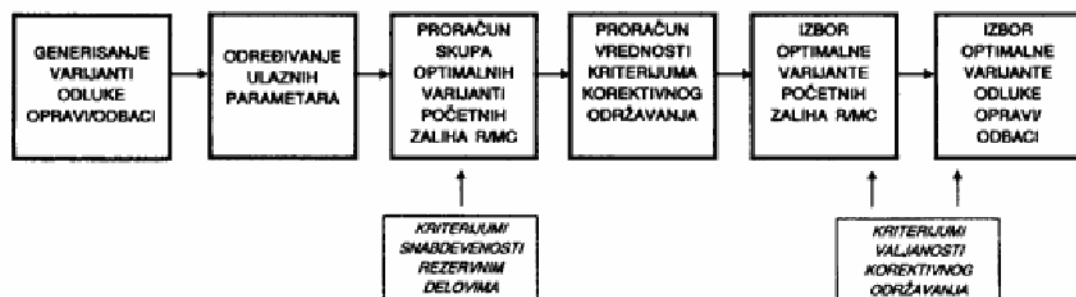
Sl. 3 — Postupak donošenja optimalne odluke opravi-odbaci
