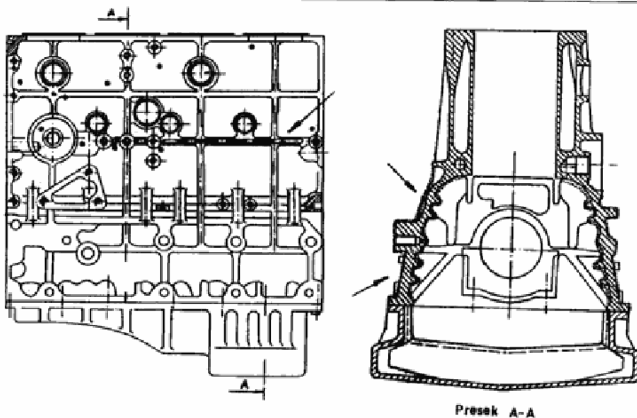
Sl. 8 - Konstrukcija bloka motora sa produženim bočnim stranicama i dodatnim orebrenjima
