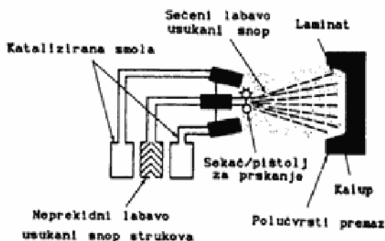
Sl. 4 – Metod prskanja u oblikovanju kompozitnih materijala
