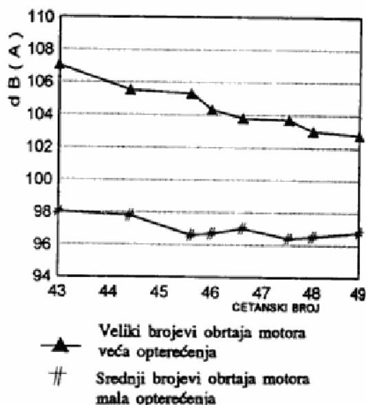
Sl. 2 - Zavisnost buke motora od cetanskog broja
