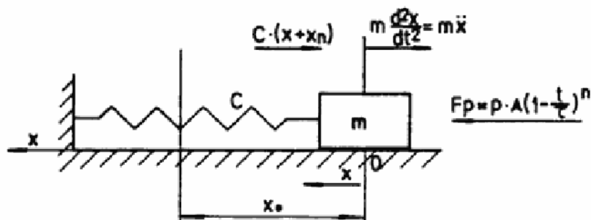
Sl. 2 – Mehanički model protivudarnog ventila
