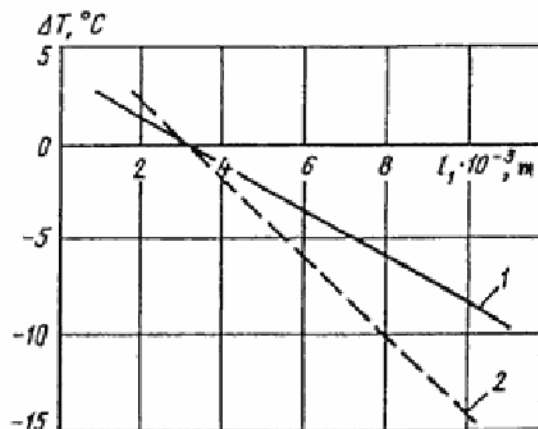
Sl. 8 – Zavisnost temperature na suprotnim stranama oblikovanog priprema, pri brzinama zagrevanja 3°C/min (1) i 8°C/min (2)
