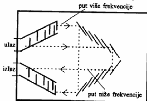
Sl. 5 - SAW čirp-linija za kašnjenje sa refleksijom zvučnog talasa
