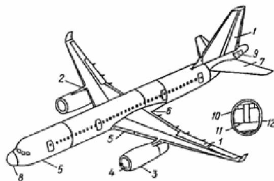
Sl. 1 – Kompozitni materijali u konstrukciji aviona Tu-204
