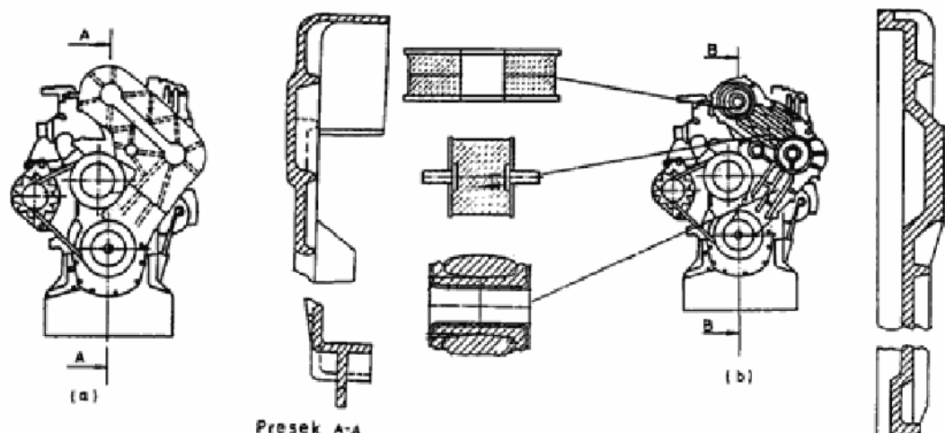
Sl. 11 – Poklopci razvoda motora: a) – plastični, b) – metalni
