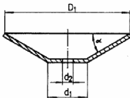
Sli. 3 – Membrana protivudarnog ventila
