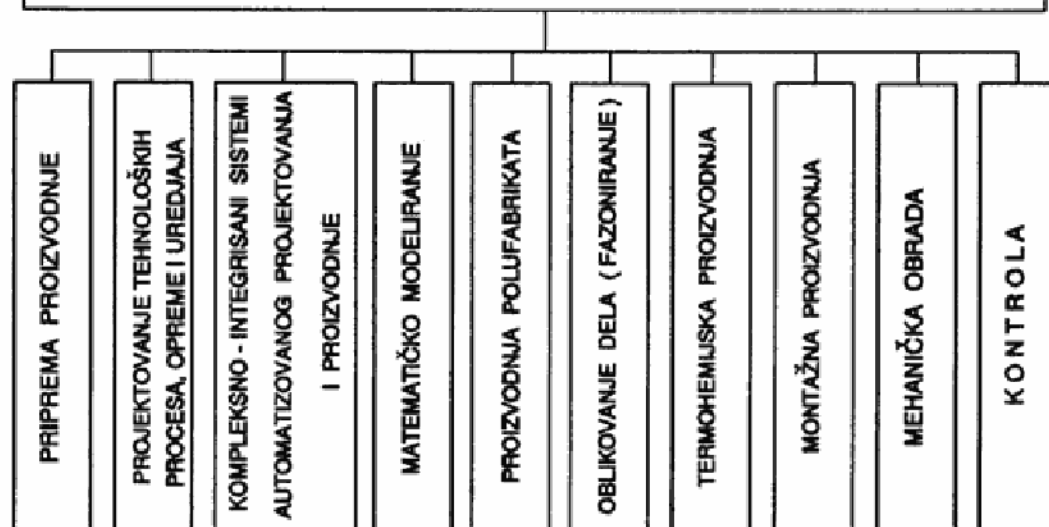
Sl. 9 – Šematski prikaz strukture proizvodnje avionskih konstrukcija od kompozitnih materijala
