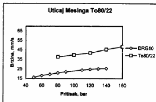
Sl. 3 – Prikaz brzina gorenja goriva DRG10 bez provodnika i sa metalnim provodnikom od mesinga
