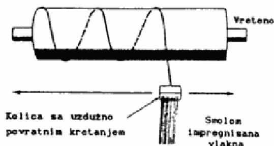
Sl. 6 – Postupak namotavanja filamenata
