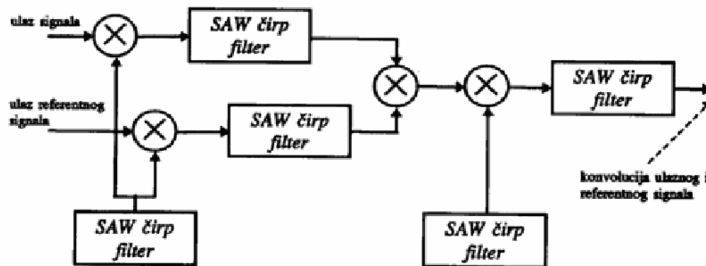
Sl. 10 – Blok-šema programabilnog filtera
