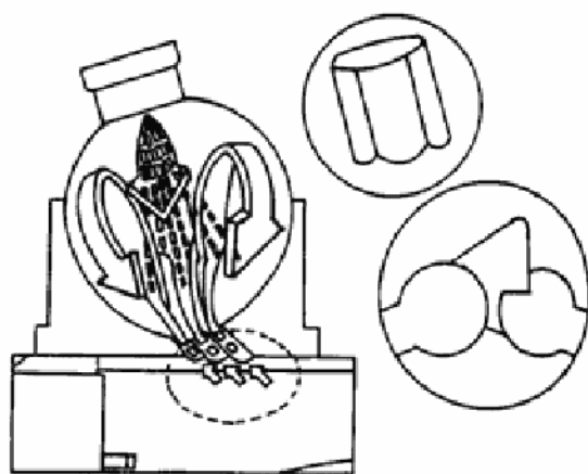
Sl. 4 – „Tvrđovrtložno“ ustrujavanje vazduha u vihornu komoru
