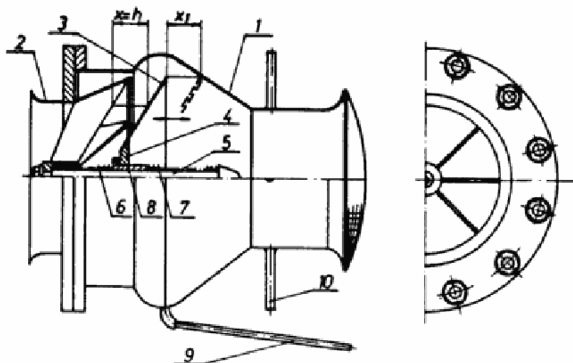
Sl. 1 – Protivudarni ventil:
