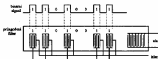
Sl. 13 – Prilagođeni SAW filter za binarni signal
