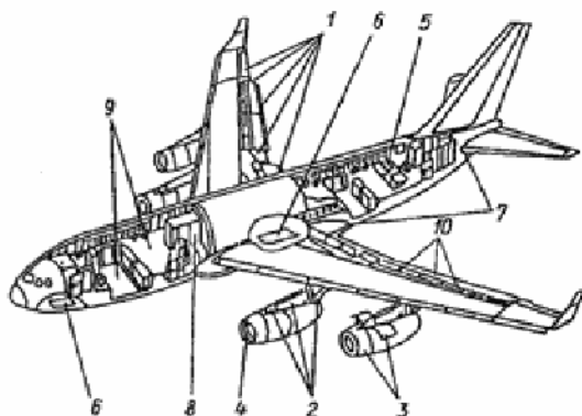
Sl. 2 – Kompozitni materijali u konstrukciji aviona Il-96-300
