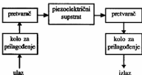
Sl. 2 – Osnovni elementi SAW komponente
