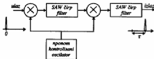
Sl. 11 – Blok-šema promenljive linije za kašnjenje
