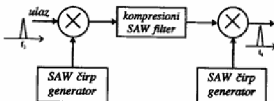
Sl. 7 – Blok-šema kompresivnog prijemnika
