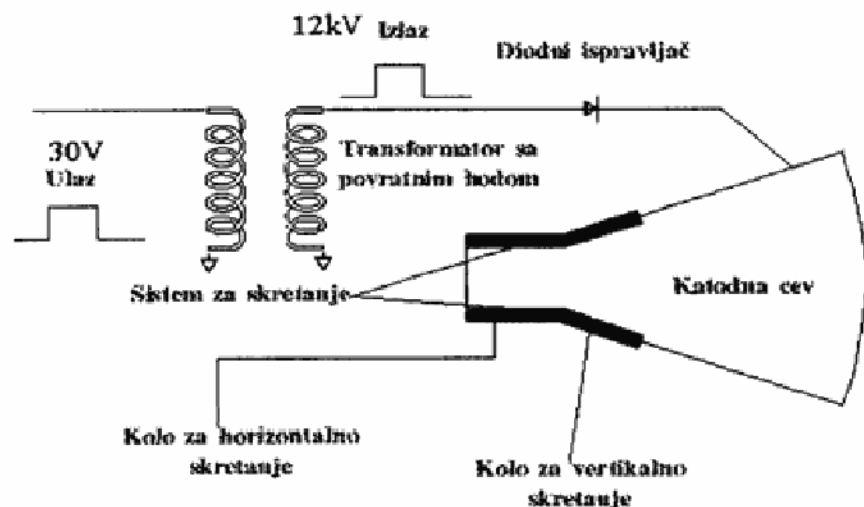
Sl. 2 – Presek video displej terminala
