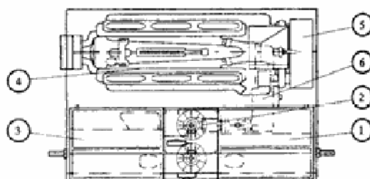
Sli. 5 – Modularna pogonska grupa: 1 i 3 – bočni menjači, 2 – ventilator, 4 – pogonski motor, 5 – prečistač vazduha, 6 – multiplikator
