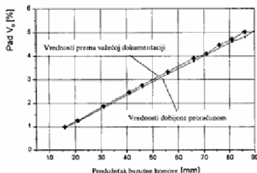
Slika 4 – Pad početne brzine projektila u zavisnosti od produžetka barutne komore za haubicu 122 mm D30J
