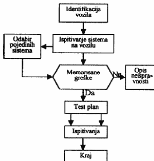
Sli. 6 – Algoritam funkcionisanja VW testera
