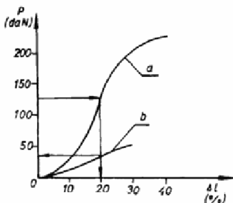
Sl. 6 – Dijagrami izduženja: a) – vrpce b) – tkanine
