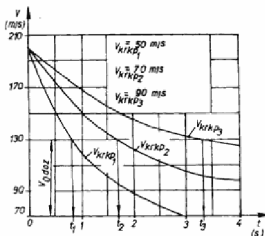
Sl. 8 – Promena vremena kočenja sistema teret-padobran do brzine V_{0, doz} u funkciji površine kočjećeg padobrana V_{kr, kp}
