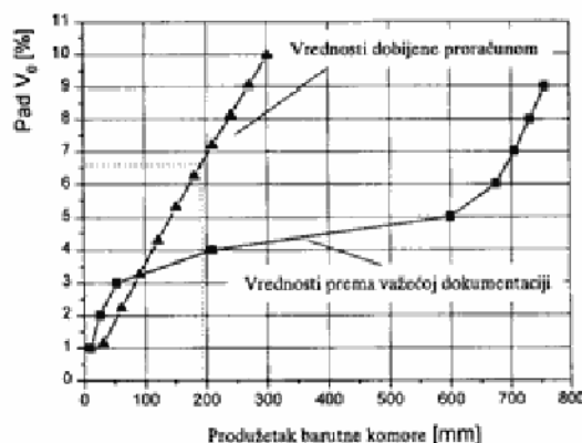
Slika 5 – Pad početne brzine projektila u zavisnosti od produžetka barutne komore za top 130 mm M46
