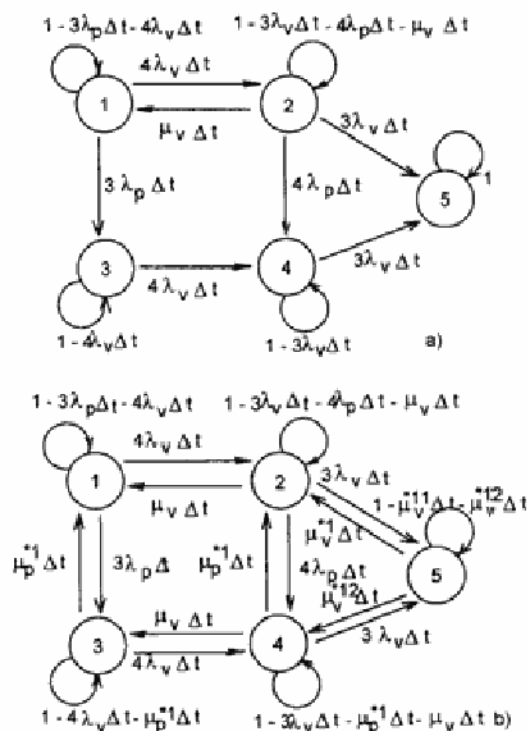
Sl. 6 – Konačan grafički prikaz modela Markova za: a) pouzdanost sistema, b) raspoloživost sistema
