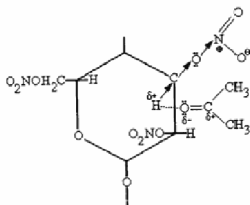
Sl. 1 – Delovanje želatinizatora ketonskog tipa na nitrocelulozu
