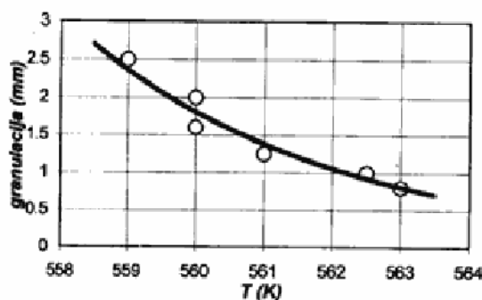
Sl. 7 – Uticaj granulacije na temperaturu paljenja kod TNT-a
