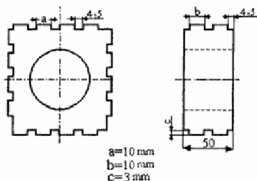
Slika 5 – Izgled uzorka DRG sa urađenim epruvetama za smicanje DRG u pravcu presovanja
