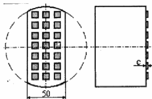
Slika 6 – Izgled uzorka sa epruvetama za smicanje čeonih inhibitora
