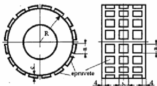
Slika 4 – Izgled uzorka (pogonskog punjenja ili segmenta pogonskog punjenja), spolja bočno inhibiranog, sa urađenim epruvetama za smicanje
