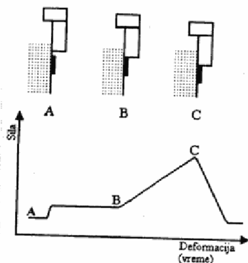
Sl. 7 – Izgled dijagrama sila–deformacija (vreme)
