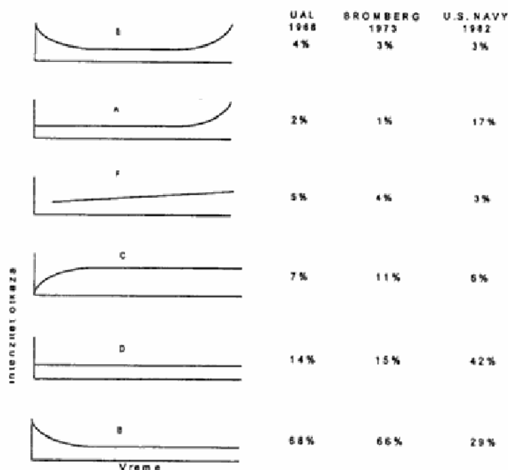
Sl. 3 – Oblici krive intenziteta otkaza
