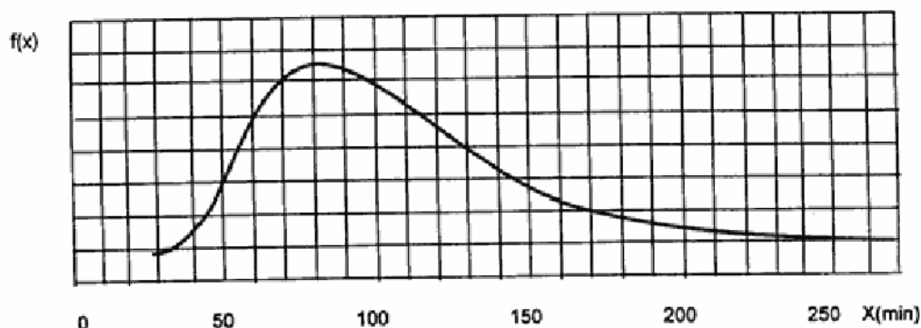
Sli. 2 - Funkcija gustine lognormalne raspodele za korektivno održavanje do nivoa komponenti
