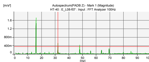
Sl. 10 – Autospektar u opsegu do 100 Hz izmerenih vibracija u pravcu z ose na mernom mestu „kod padobranca“ pri horizontalnom letu brzinom od 225 km/h
