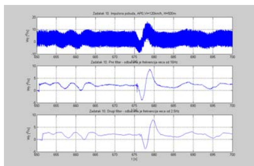
Sl. 7 – Ugaona brzina po Y osi tokom izvođenja manevra
