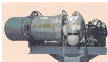
Slika: Sistem MANTA DIRCM za odbranu aviona od prenosnih raketa PVO
