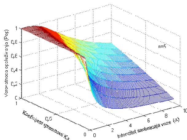
Slika 6 – Zavisnost verovatnoće opsluživanja od koeficijenta spremnosti i intenziteta saobraćaja veze
