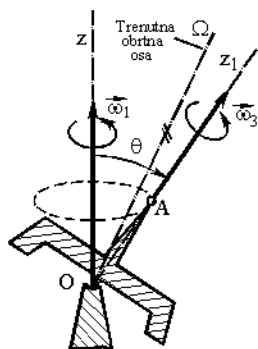
Slika 1 – Žiroskop
