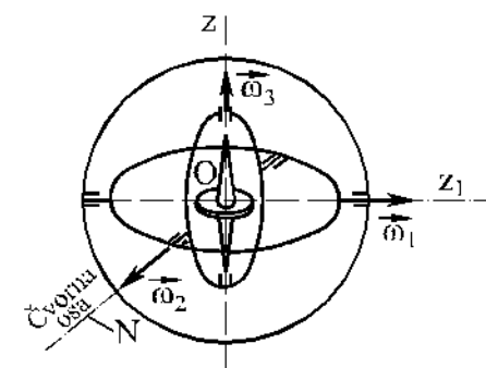
Slika 2 – Žiroskop u kardanovom ramu
