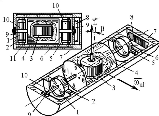
Slika 12 – Plivajući žiroskop
