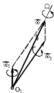
Slika 1 – Žiroskop
