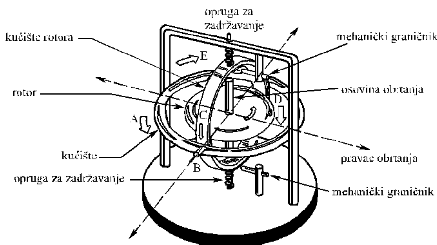
Slika 23 – Dejstvo brzinskog žiroskopa
