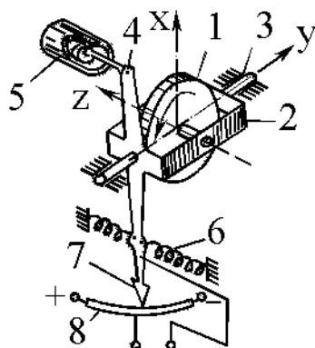
Slika 22 – Brzinski žiroskop
