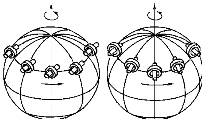
Slika 19 – Ponašanje slobodnog žiroskopa tokom rotacije Zemlje
