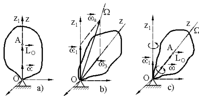
Slika 3 – Telo pri sfemnom kretanju
