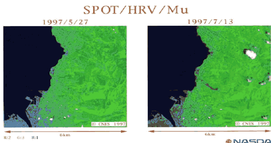
Slika 10 – Stereo par HRV, SPOT snimaka [2]
