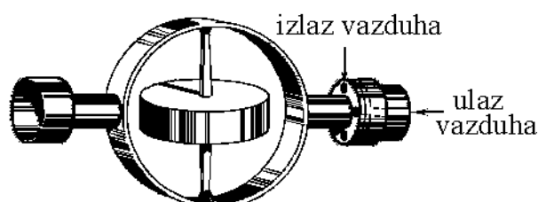
Slika 13 – Žiroskop sa vazdušnim ležajima
