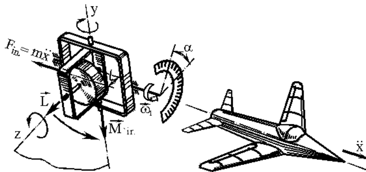
Slika 25 – Šema i princip rada žiroskopa za merenje linearne brzine
