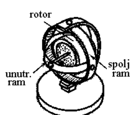
Slika 28 – Mehanički brzinski žiroskop sa dva stepena slobode
