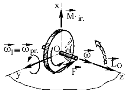
Slika 16 – Pravilo precesije
