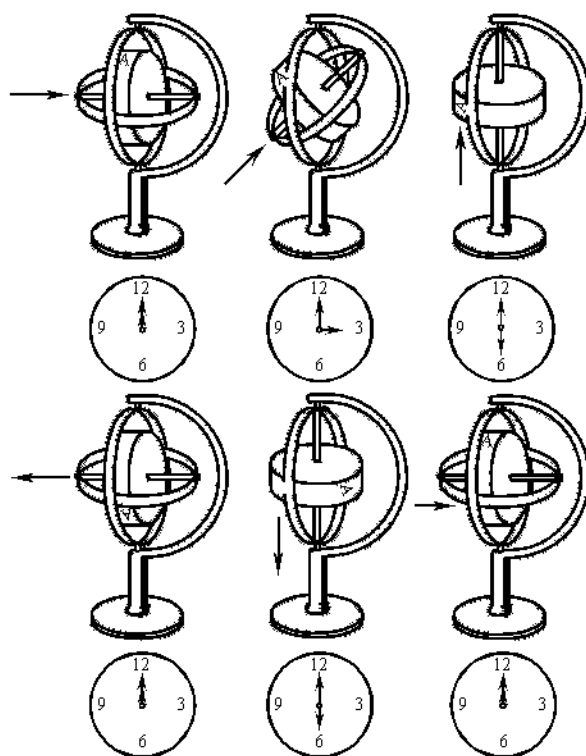
Slika 21 – Prividna precesija
