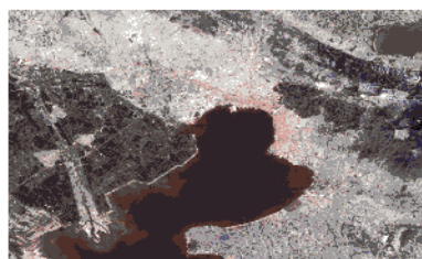
Slika 5 – Snimak Soluna načinjen tematskim maperom sa satelita Landsat [6]
