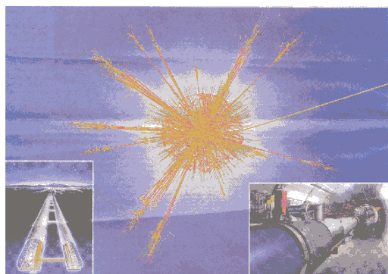
Velika slika: Otisak u sudaru protonskih mlazeva
