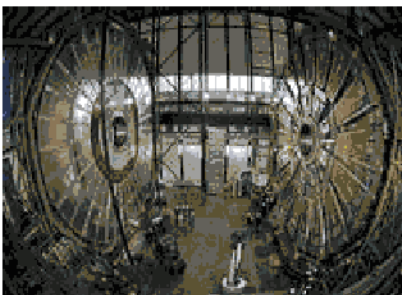
Detektor CMS na LHC-u
