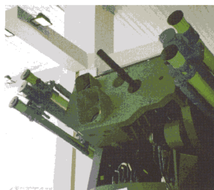
Slika: Postolje turskog sistema PVO Aselsan sa 4 rakete Igla
