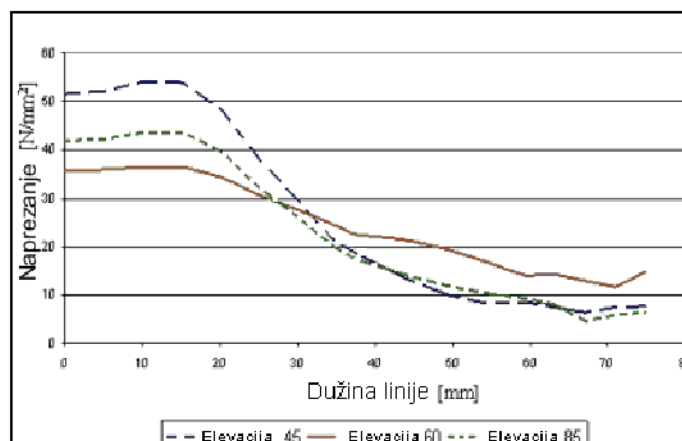
Slika 7 – Dijagram naprežanja materijala po liniji koja sadrži merno mesto I
