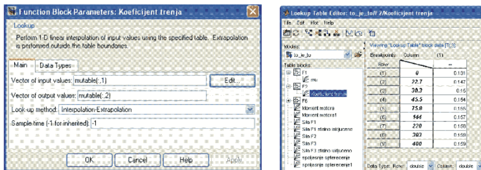
Slika 10 – Koeficijent trenja u funkciji brzine klizanja
