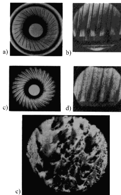
Slika 1 – Oštećenja površine cevi oruđa 105 mm M68 kao rezultat opaljenja metka:
