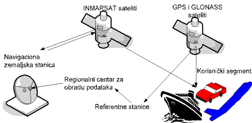
Slika 1 – Sistem WAAS
