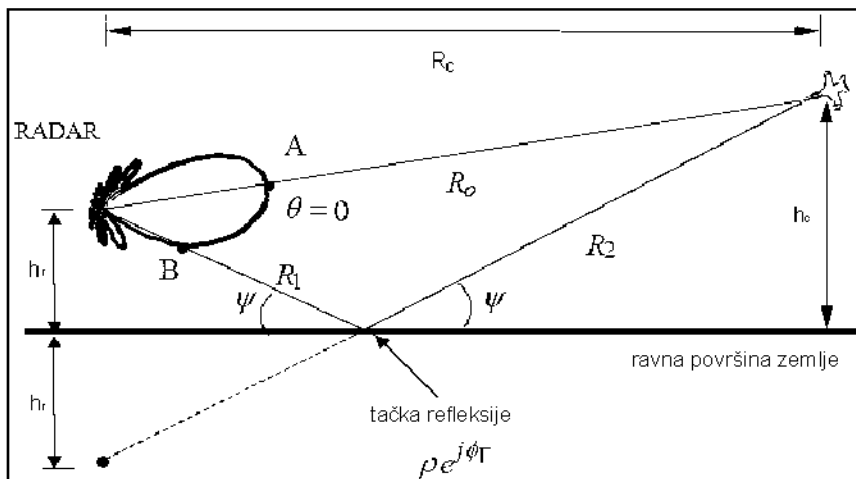
Slika 3 – Refleksija signala sa ravnog tla
