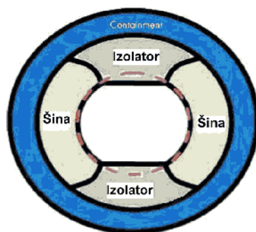
Slika 9 – Izgled preseka cevi šinskog EM topa [17]
