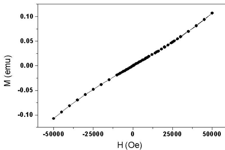
Slika 12 – Zavisnost magnetnog dipolnog momenta od magnetnog polja za uzorak hematita visokog kristaliniteta na temperaturi 100 K
