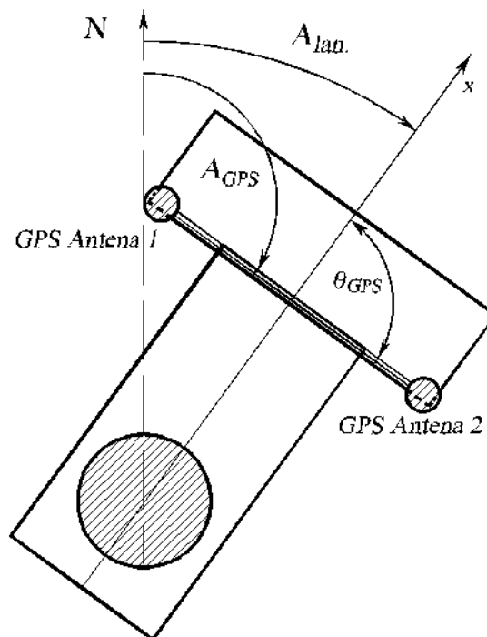
Slika 7 – Orijentacija pomoću GPS prijemnika sa dve antene Figure 7 – Orientation using a GPS receiver with two antennas
