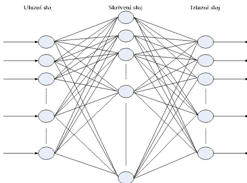
Slika 6 – Višeslojna neuronska mreža
