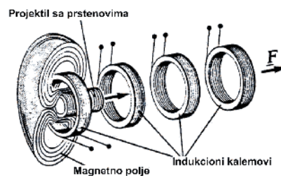
Slika 2 – Funkcionalna šema solenoidnog EM topa
