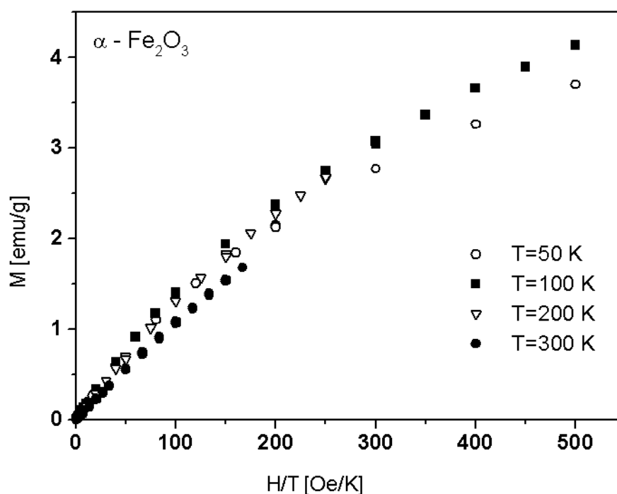
Slika 7 – Zavisnost magnetizacije od H/T Figure 7 – Magnetization of \alpha -Fe 2 O 3 nanoparticles as a function of H/T
