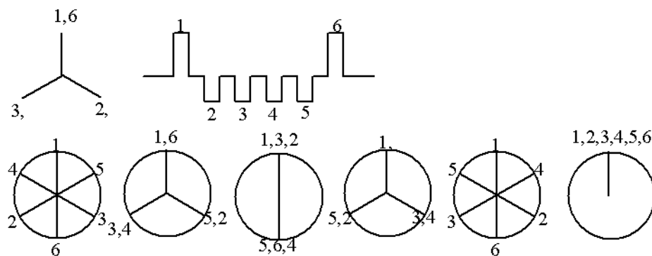
Slika 5 – Raspored kolena četvorotaktnog šestocilindričnog linijskog motora i fazni dijagram harmonika pobudnog momenta
