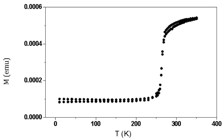
Slika 11 – Zavisnost magnetnog dipolnog momenta od temperature za uzorak hematita visokog kristaliniteta u magnetnom polju jačine 100 Oe (ZFC i FC merenja)
