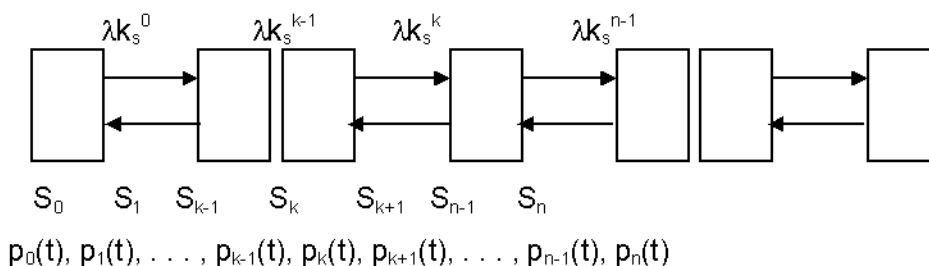
Slika 2 – Prikaz grafa stanja sistema
