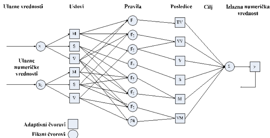
Slika 7 – Opšta struktura adaptivne neuro-fuzzy mreže
