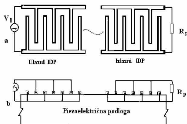
Slika 2 – Šematski prikaz transversalnog PAT filtera tipa linije za kašnjenje
