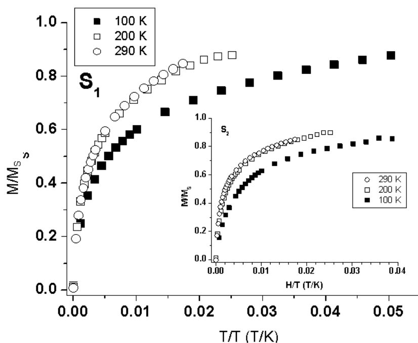
Slika 9 – Zavisnost M/M_s od H/T za uzorke nanočestićnog maghemita Figure 9 – Dependence M/M_s on the H/T for the nanoparticle \gamma\text{-Fe}_2\text{O}_3
