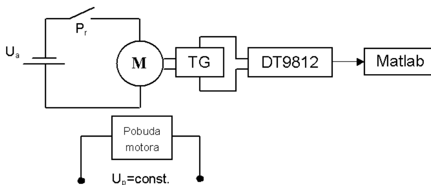
Slika 5 – Principialna šema za identifikaciju jednosmernog motora Figure 5 – Principle chart for the identification of DC motors
