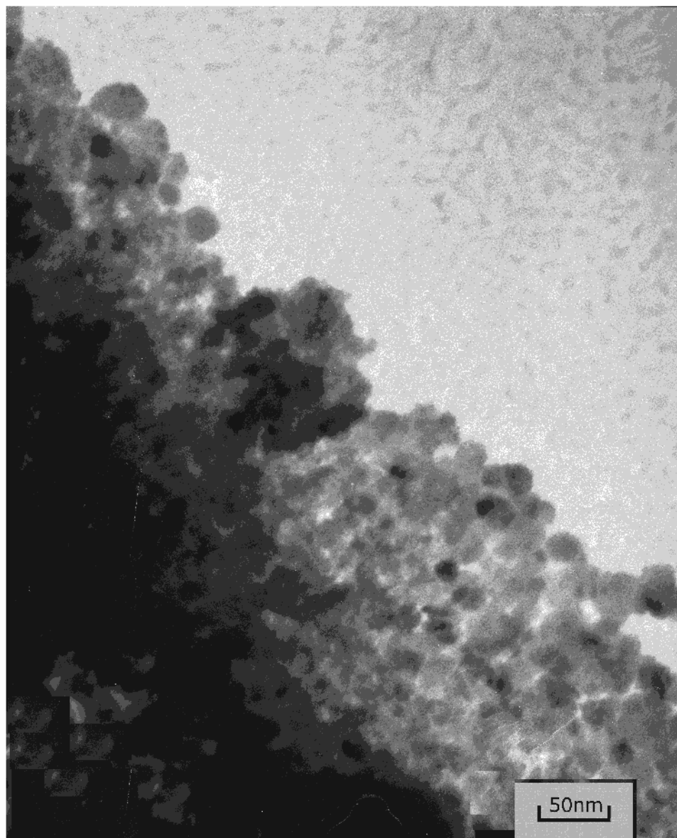
Slika 3 – Fotografija dobijena pomoću TEM-a za uzorak S_2 nanočestičnog \gamma\text{-Fe}_2\text{O}_3
