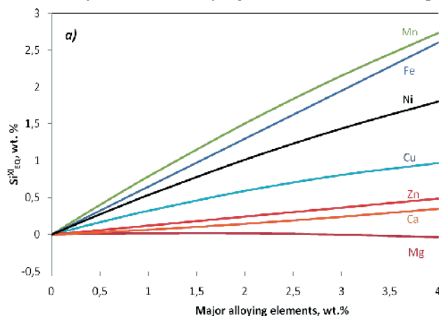
Figure 3 a - The effect of major alloying elements on the Si_{EQ}^{Xi} for hypoeutectic alloys Slika 3 a - Uticaj glavnih legirajućih elemenata na Si_{EQ}^{Xi} za hipotetičke legure
