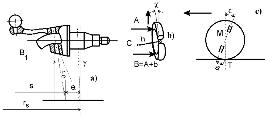
Slika 4 – Šematski prikaz parametara geometrije oslanjanja desnog prednjeg točka Figure 4 – Schematic view of the suspension geometry parameters of the right front wheel
