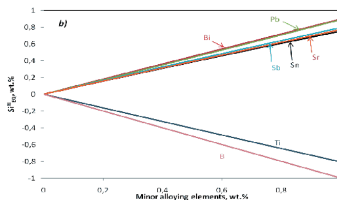
Figure 3 b - The effect of minor alloying elements on the Si_{EQ}^{Xi} for hypoeutectic alloys. Slika 3 b - Uticaj minornih legirajućih elemenata na Si_{EQ}^{Xi} za hipotetičke legure
