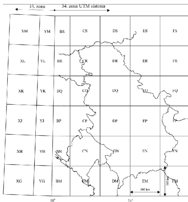
Slika 9 – Podela i označavanje kvadrata 100 \times 100 km UTM mreže Figure 9 – UTM grid of area 100 \times 100 km
