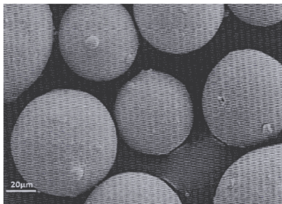
Figure 2 - (SEM) Scanning electron micrograph of the NiCrBSi powder particles Slika 2 - (SEM) Skenirana elektronska mikrofotografija čestica praha NiCrBSi
