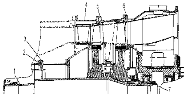
Slika 7 – Turbina visokog pritiska
