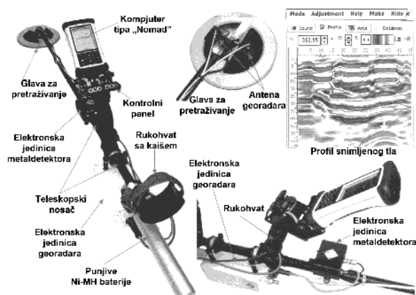
Sastavni delovi detektora metala „mirador“
