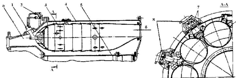
Slika 5 – Komora sagorevanja
