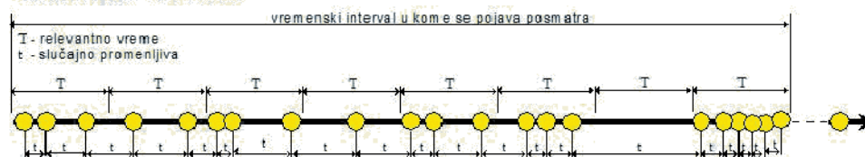
Slika 1 – Prikaz stohastičkog vremena između dva zahteva
